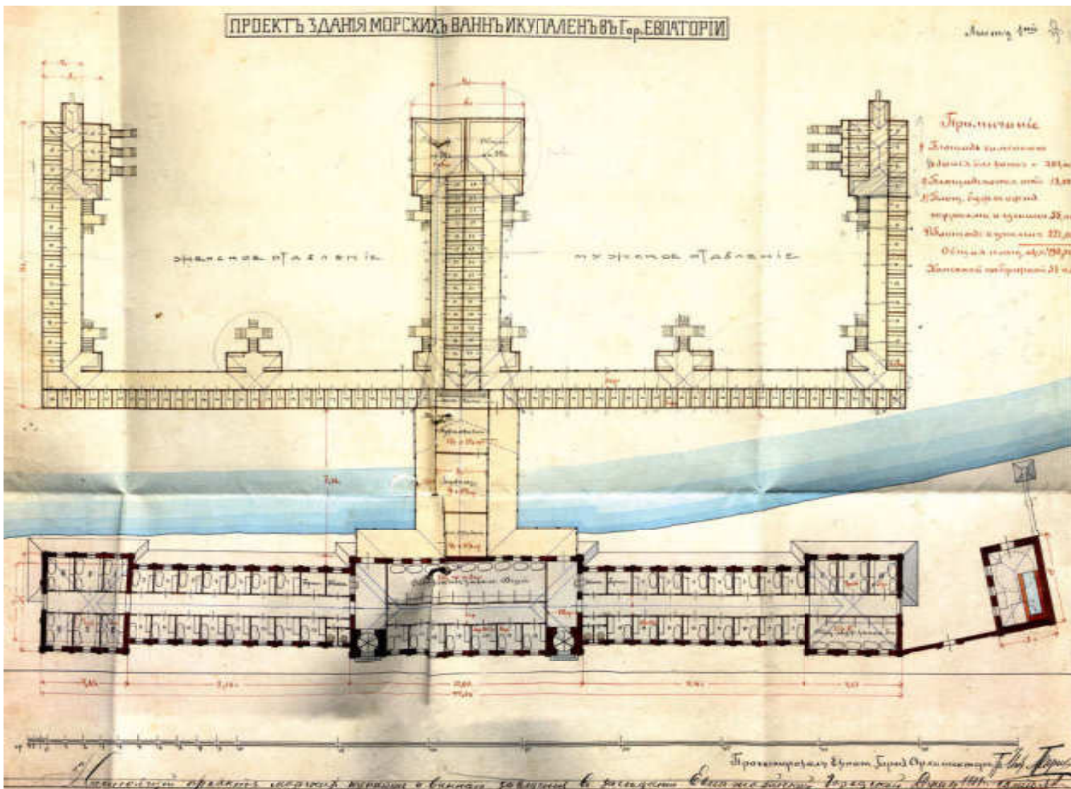
Адам Генрих. Проект здания морских ванн и купален в г. Евпатории. Государственный архив Республики Крым
