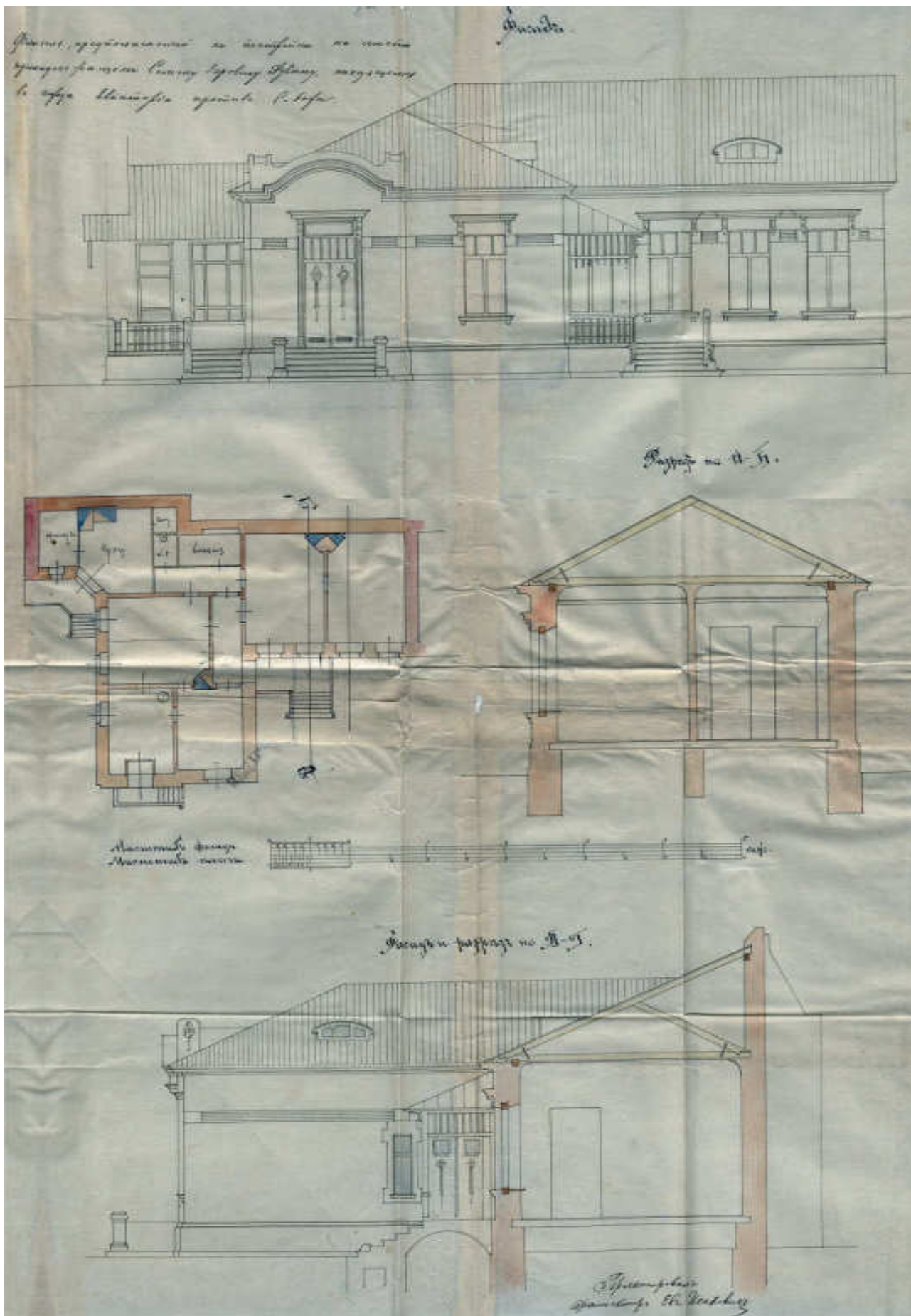
Е.С. Исакович. Проект флигеля, принадлежавшего С.Э. Дувану. Государственный архив Республики Крым
