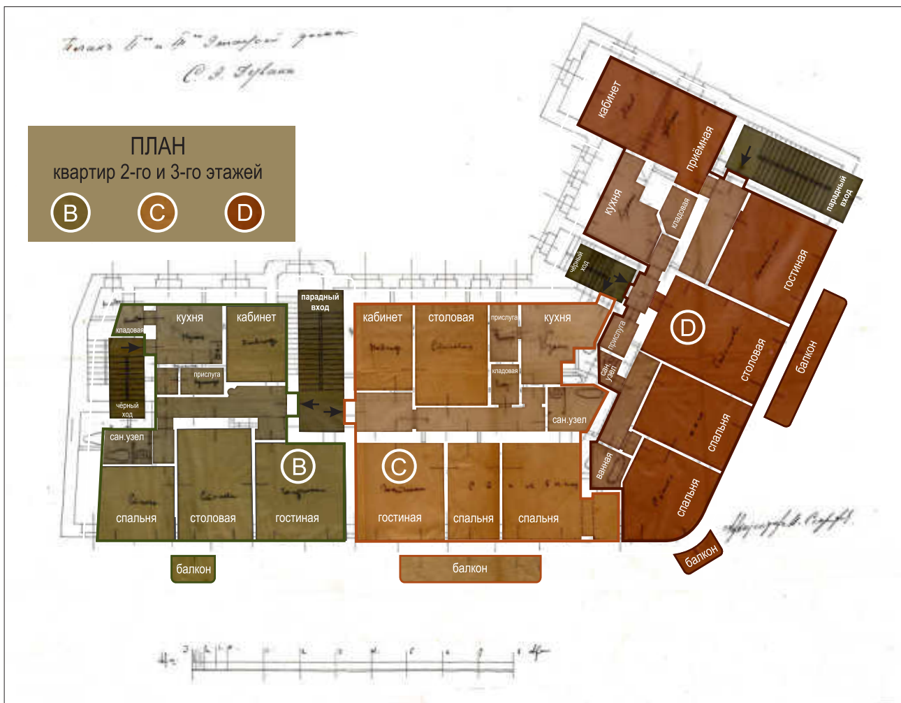
Поэтажные планы Дома Дувана. Моделирование на основе плана П.Я. Сеферова: Татьяна Савченко
