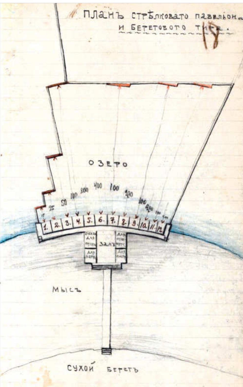
План стрелкового павильона и берегового тира. Российский государственный военный архив
