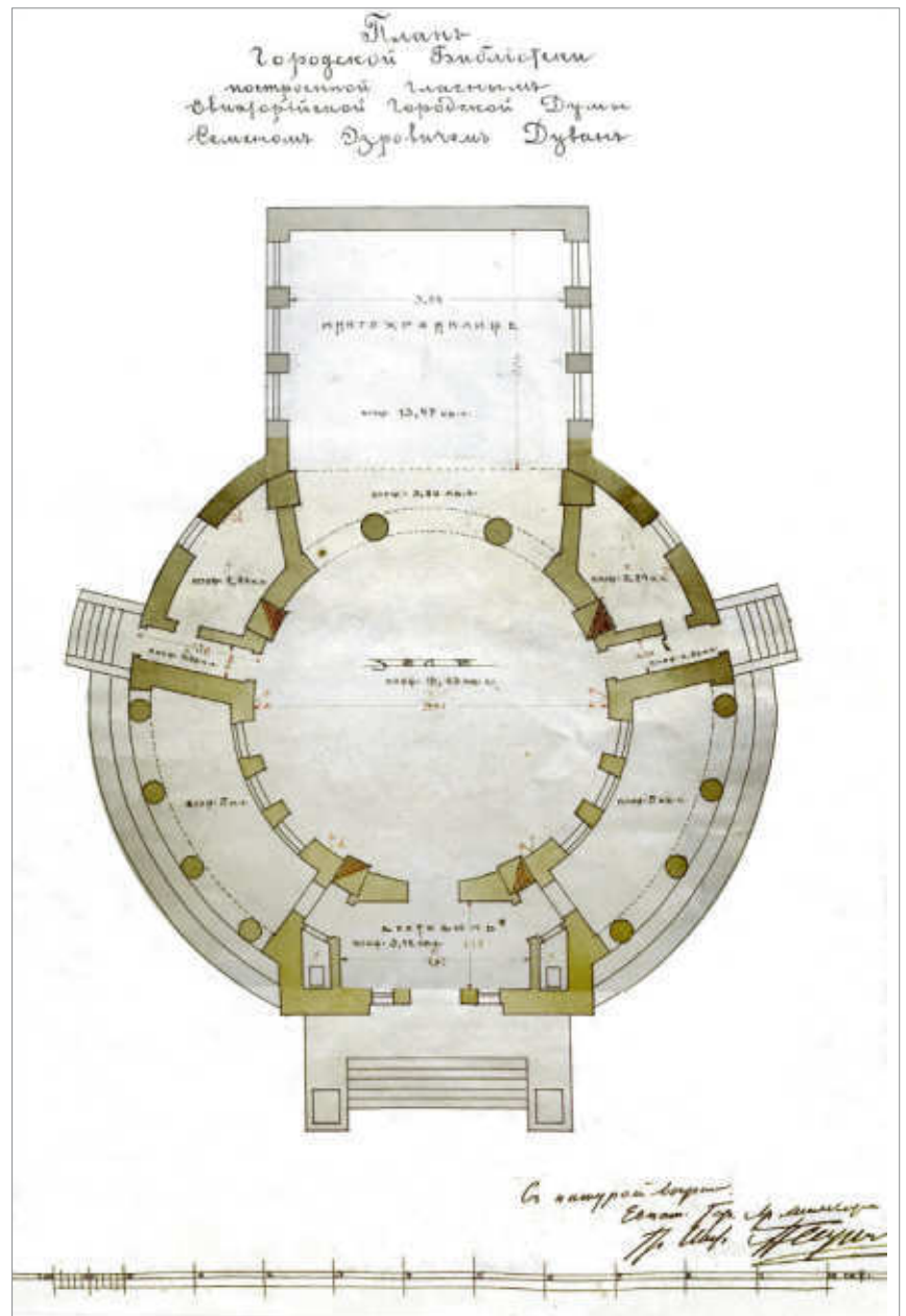
План библиотеки. Евпаторийский краеведческий музей
