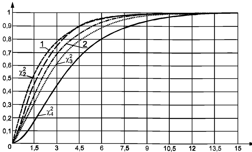
Рисунок 7 — Распределение статистики S_{\text{он}} при пяти интервалах группирования и оценивании двух параметров нормального распределения
