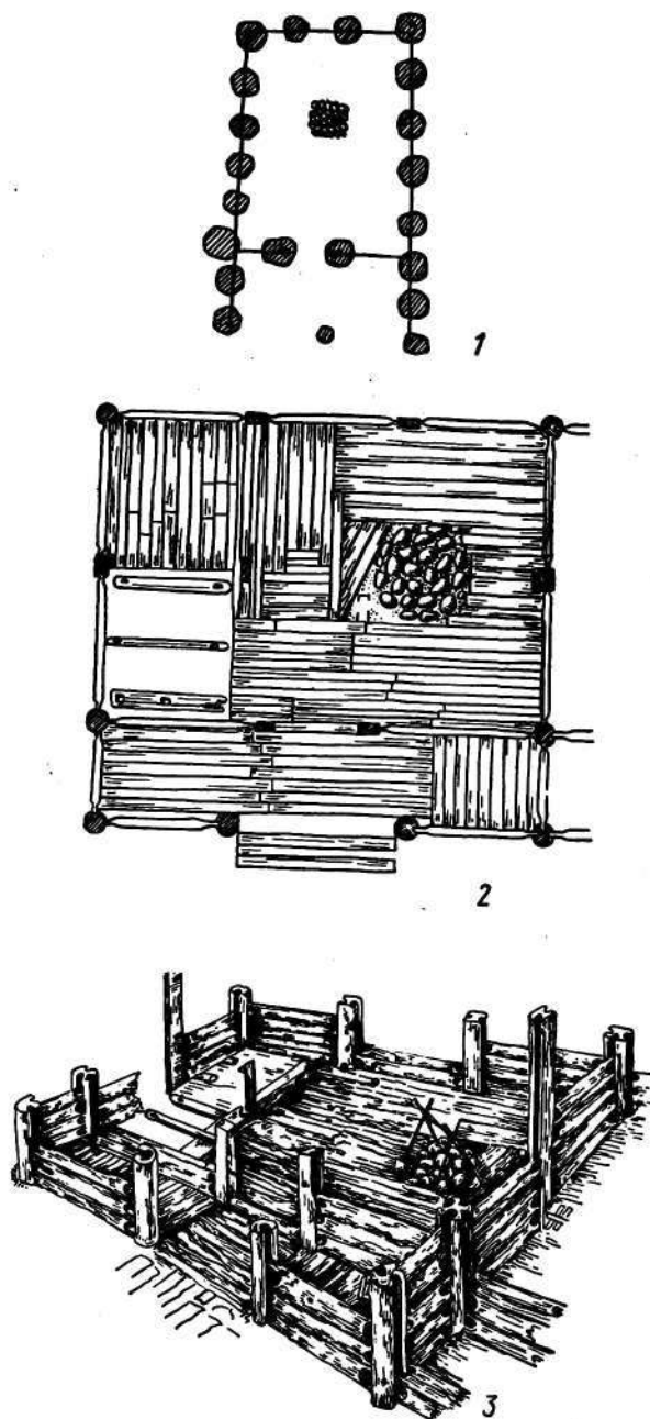
Рис. 53. Жилища ЛУЖИЦКОЙ КУЛЬТУРЫ: 1 — план дома-мегагона в Ремершанце, 2 — план жилища Бискупинского городища, 3 — конструкция дома Бискупинского городища
