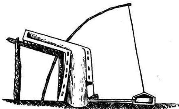
Р и с . 2. НАГНЕТАНИЕ ВОЗДУХА В СЫРОДУТНЫЙ ГОРН
