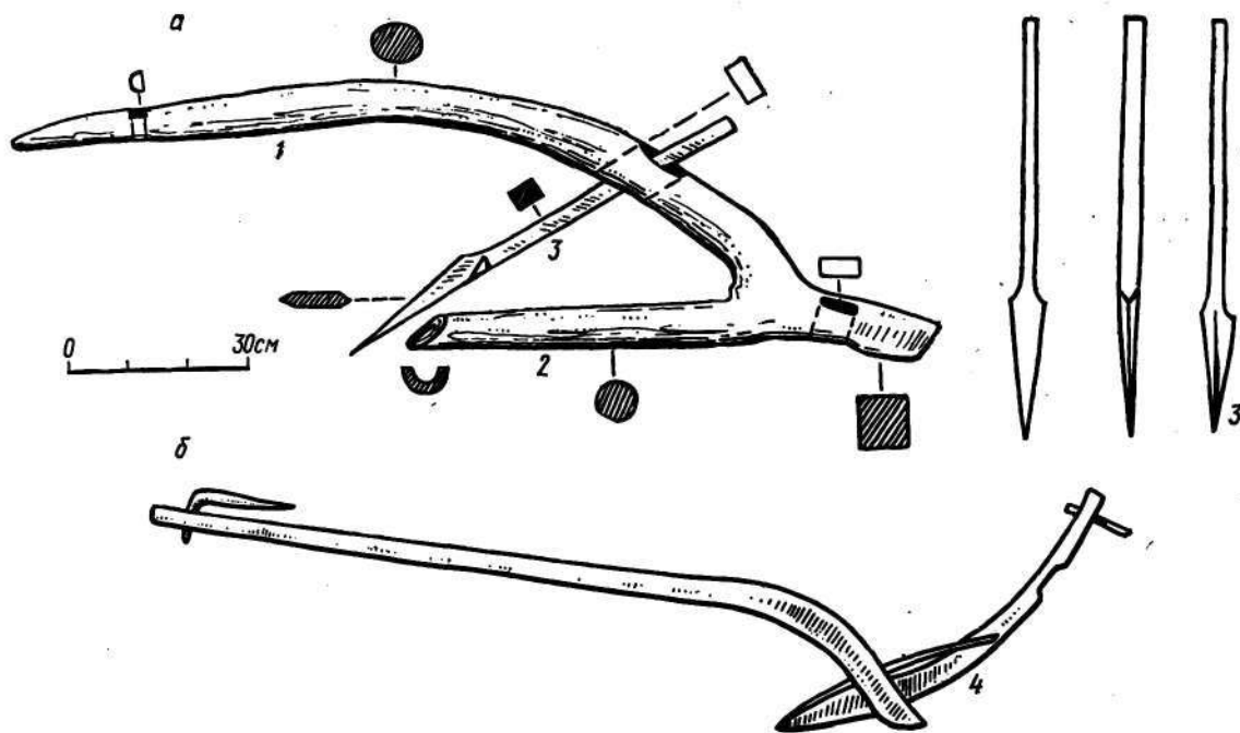
Рис. 29. ПЛУГИ ГАЛЬШТАТСКОГО ВРЕМЕНИ: а — Дабергготц, б — Деструп; 1 — грядиль, 2 — ползун, 3 — резак, 4 — сошник
