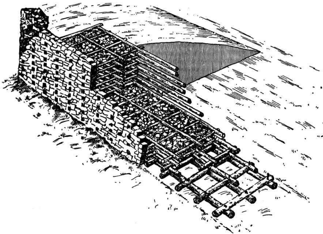
Рис. 35. КОНСТРУКЦИЯ КЕЛЬТСКОЙ КРЕПОСТНОЙ СТЕНЫ (по Ж. Дешелетту)
