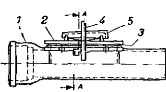
Anma boyutu 100 olan A biçiminde kır döküm ve kır döküm köprü tü temizleme borusunun gösterilişi: Temizleme borusu A KD 100 TS 10/21
