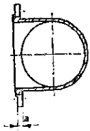
Anma boyutu 100 olan bir temizleme borusunun gösterilişi: Temizleme borusu 100 TS 10 / 20
