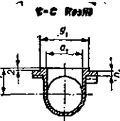
Anma boyutu 100 olan kır döküm temizleme borusunun gösterilişi: Boru 100 TS 10 / 21
