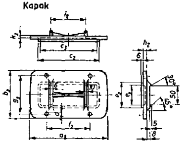
Anma boyutu 100 olan kır döküm bir temizleme borusu kapağının gösterilişi: Kapak 100 TS 10 / 21
