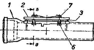
Anma boyutu 100 olan B biçiminde (civatabağlantılı) temizleme borusunun gösterilişi:
