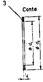
Anma boyutu 100 olan bir temizleme borusu kapak contasının (lâstik) gösterilişi. Conta 100 TS 10 / 20
