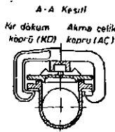
Anma boyutu 100 olan A biçiminde kır döküm ve kır döküm köprü tü temizleme borusunun gösterilişi: Temizleme borusu A KD 100 TS 10/21
