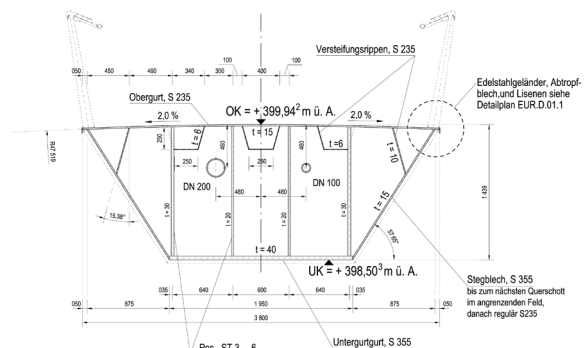
Brückenquerschnitte in Feldmitte (unten) sowie am Auflager (oben)
