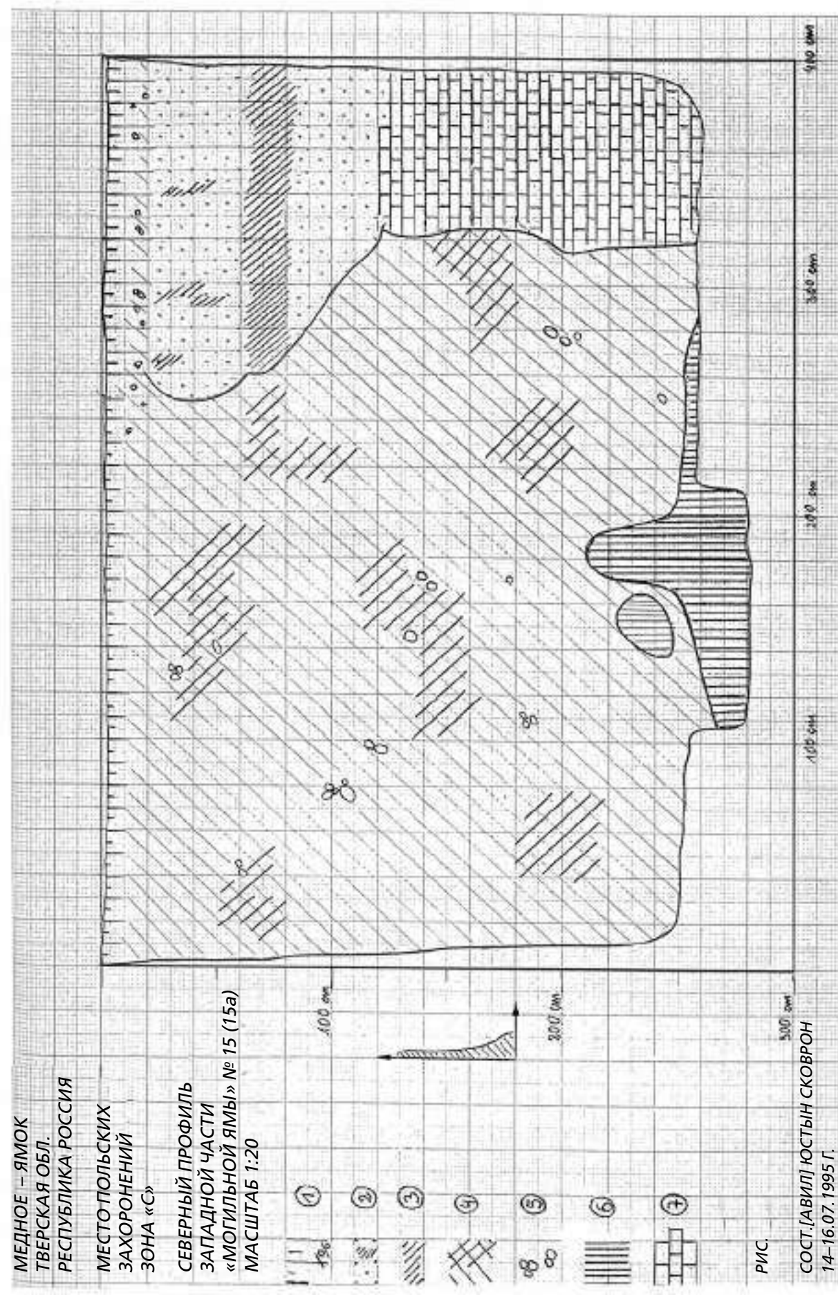
[Геологический профиль могильной ямы № 15а.
