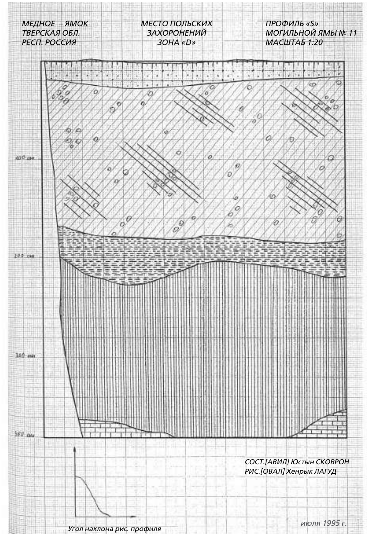
[Геологический профиль могильной ямы № 11. Условные обозначения объяснены на последней странице тома III отчета (см. ниже с. 650)]
