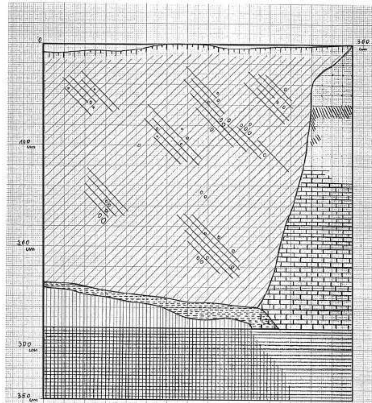
MIEDNOJE - JAMOK OBL. TWERSKA REP. ROSJA MIEJSCE POCHÓWKÓW POLSKICH STREFA "C" PROFIL "W" DOŁU ŚMIERCI NR 20 SKALA 1:20
