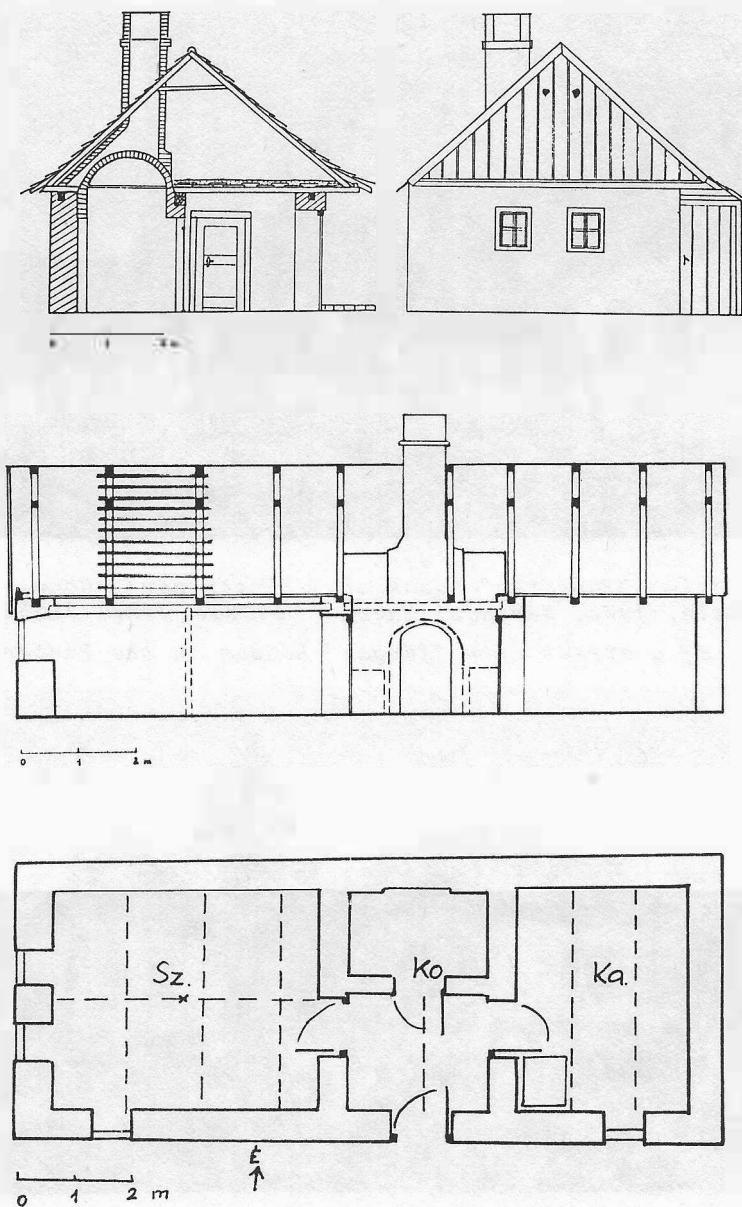
5. ábra Erdő u. 8. sz. ház felmérési rajza. H. Csukás Györgyi felmérése, 1987. Survey sketch of the house in Erdő St. 8.
