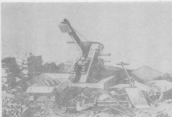
20. ábra Molnár Lajos technikus kavicsstörő gépe /F...r 1862. 329./
