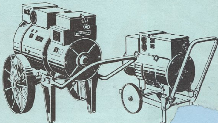
Grupos transportáveis para a soldadura eléctrica pelo em corrente continua de 80-160 A e 240-300 A
