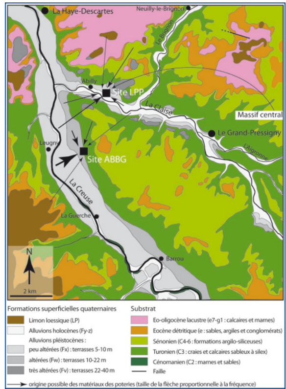
Fig. 2 : Carte géologique de la région du Grand-Pressigny (Indre-et-Loire) et provenances possibles des matériaux céramiques. D'après les cartes à 1/50000 e de Preuilly-sur-Claise (Rasplus et al. 1978) et Châtellerault (Médioni et al. 1974).
