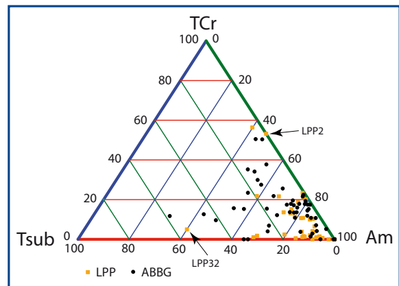
Fig. 4 : Diagramme ternaire TCr/Am/Tsub. TCr : traceurs Creuse (plagioclases, biotite, amphiboles, grenat, roches plutoniques et métamorphiques). Am : autres minéraux. Tsub : traceurs de substrat crétacé et tertiaire (= Rexo : roches sédimentaires siliceuses, glauconie et bioclastes).
