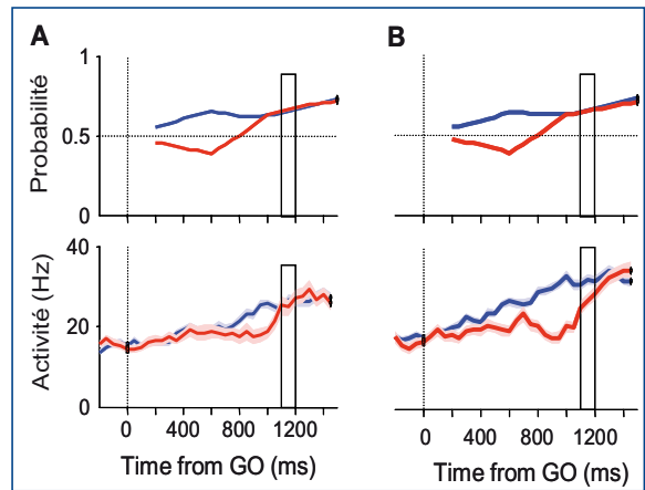
Figure 8 : Analyse ayant pour but de tester les prédictions des modèles « intégration » et « urgence » dans l'activité neuronale moyenne d'une population de cellules liées à la décision de PMd (A) et PFC (B). Panneaux du haut. Probabilité de succès dans deux types d'essais (liés aux essais « biais en faveur » et « biais en contre »). Dans les deux types d'essais, le même niveau de probabilité de succès est atteint après le 5 e déplacement de jeton, mais dans un groupe, un biais initial favorise la cible correspondant à la direction préférée des cellules (bleu) alors que dans l'autre, le biais initial favorise la cible opposée (rouge). Seuls les essais pour lesquels le singe a pris sa décision après ce biais sont inclus dans l'analyse. Panneaux du bas. Activité neuronale moyenne d'une population de cellules de PMd (n = 16, C) et PFC (n = 13, D) dans les deux groupes d'essais décrits ci-dessus. Les cadres illustrent la période critique d'analyse pour la distinction des deux modèles.
