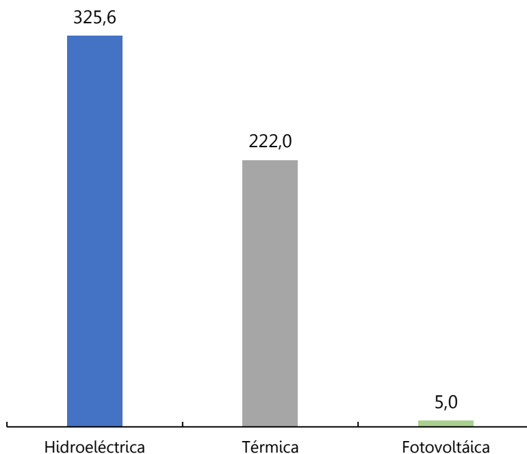
Gráfico 38. Potencia instalada por tipo de central (MW). 2017
