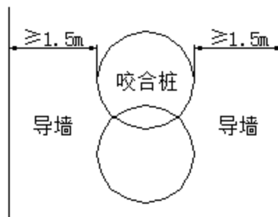
图 3-1 咬合桩两侧导墙宽度要求
