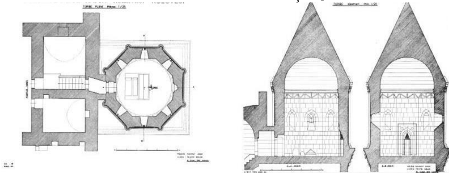
12. Huand xatun türbəsinin plan və kəsiyi.
