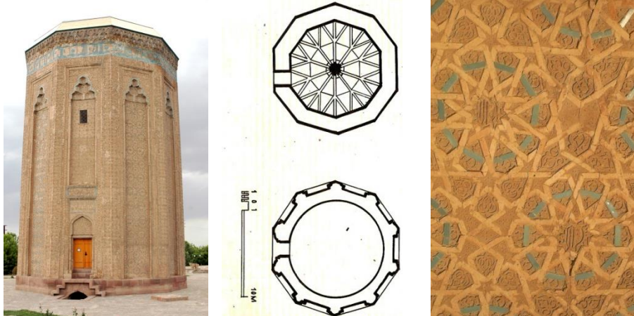
5. Kompleksə daxil olan Möminə xatun türbəsi. Türbənin sərdabə və gövdəsinin planı. Türbənin səthlərindən birinin bəzək kompozisiyası
