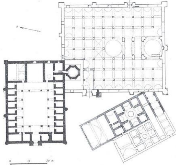
10. Huand xatun kompleksinin planı. Kayseri. (H.Karamağaralı, 1976)
