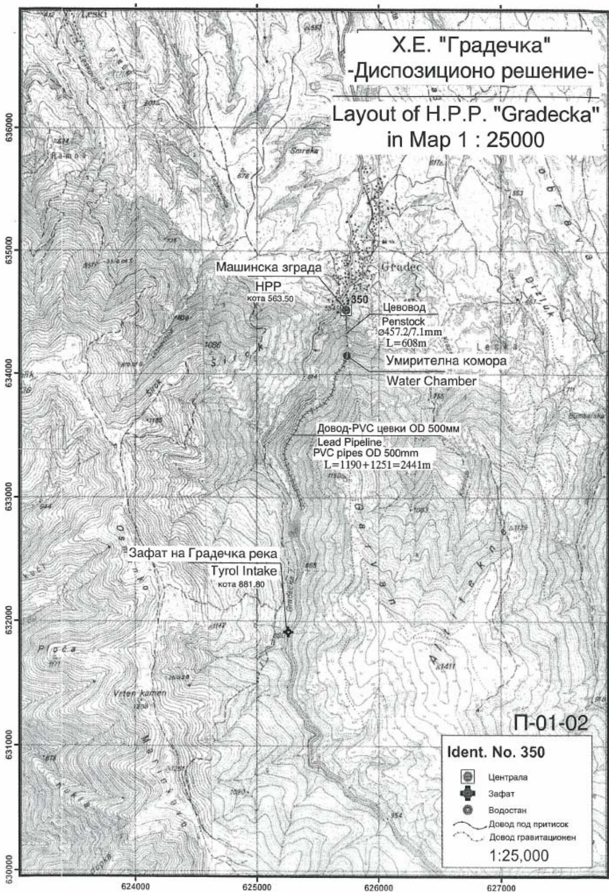
Слика – Локација на постројки и инфраструктура на МХЕ Градечка
