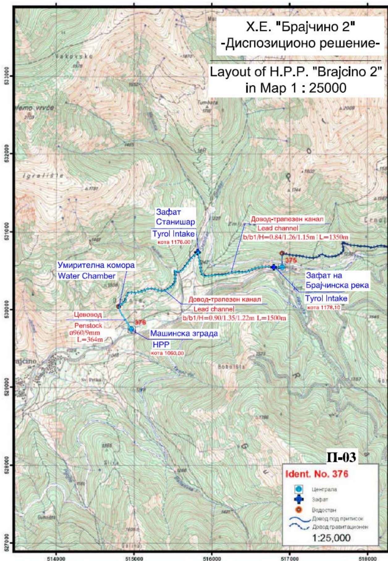
Слика – Локација на постројки и инфраструктура на МХЕ Брајчино 2
