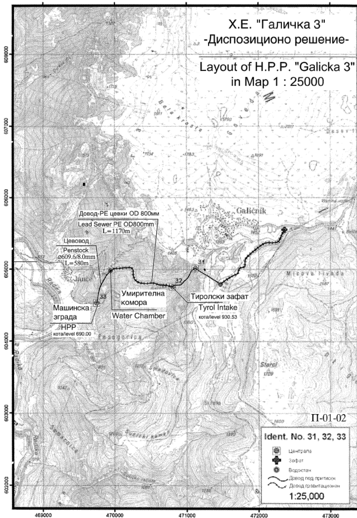
Слика – Локација на постројки и инфраструктура на МХЕ Галичник 3
