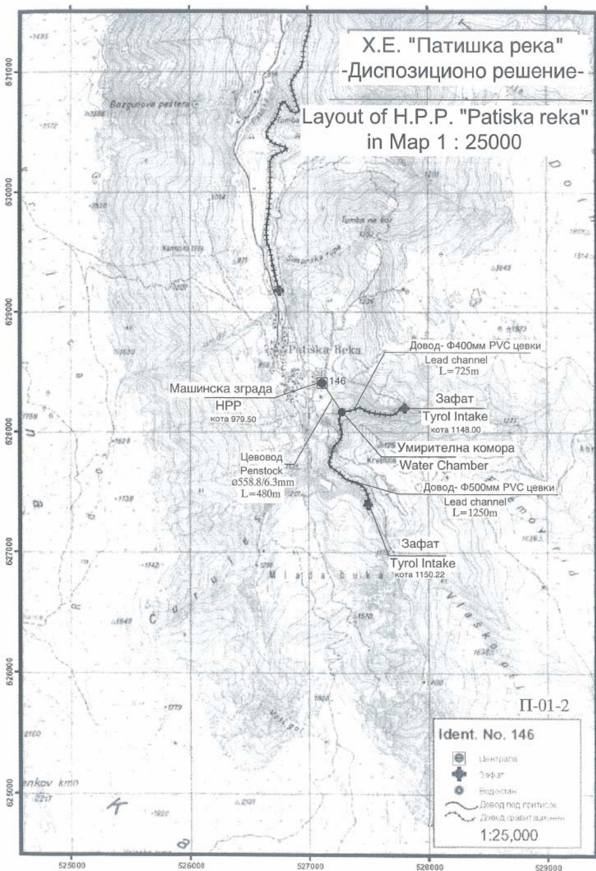
Слика – Локација на постројки и инфраструктура на МХЕ Патишка Река
