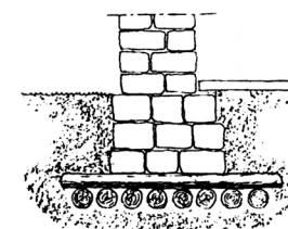
Parvele toetuv vundament. (Joonis: I. Holmström, C. Sandström "Maintenance...")
