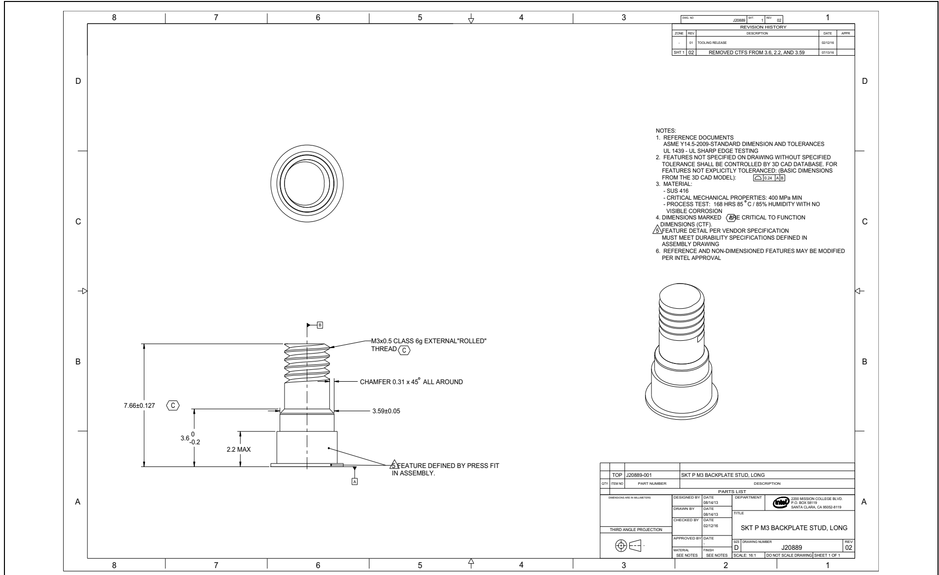
Figure D-34. Backplate Stud: Long
