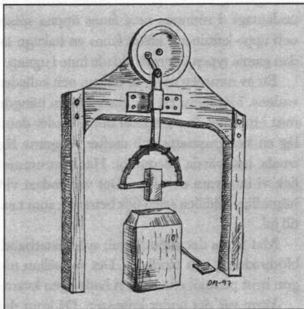
Liasmedens fjäderhammare.
