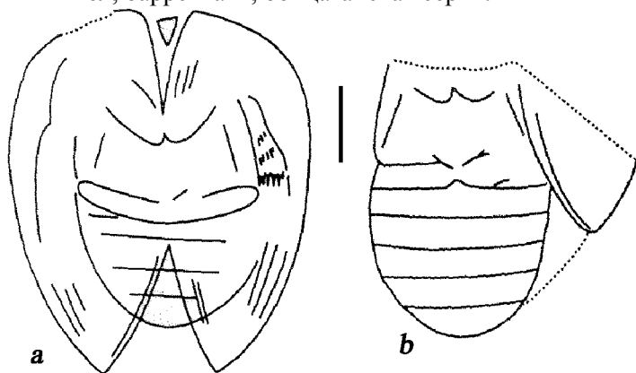
Рис. 18. Prototrox transbaikalicus Nikolajev: a – голотип ПИН № 2385/1096; b – паратип ПИН № 3559/2217. Прямая линия – 1мм [По: Николаев, 2000а]
