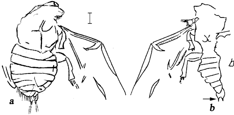
Рис. 8. Cretocoma toloigoica Nikolajev голотип ПИН, № 4271/217: a - вид сверху, b - вид снизу. Прямая линия - 1 мм [По: Николаев, 2002.]
