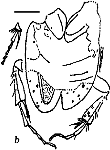
Рис. 45. Cretoscarabaeus lentiginosus Nikolajev, – голотип ПИН, № 4210/702. Прямая линия – 1мм [По: Николаев, 1995a.]
