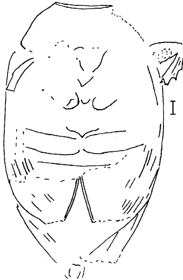
Рис. 27. Cretobolbus rohdendorfi Nikolajev, голотип ПИН, № 3064/7137. Прямая линия – 1 мм [По: Николаев, 1996].
