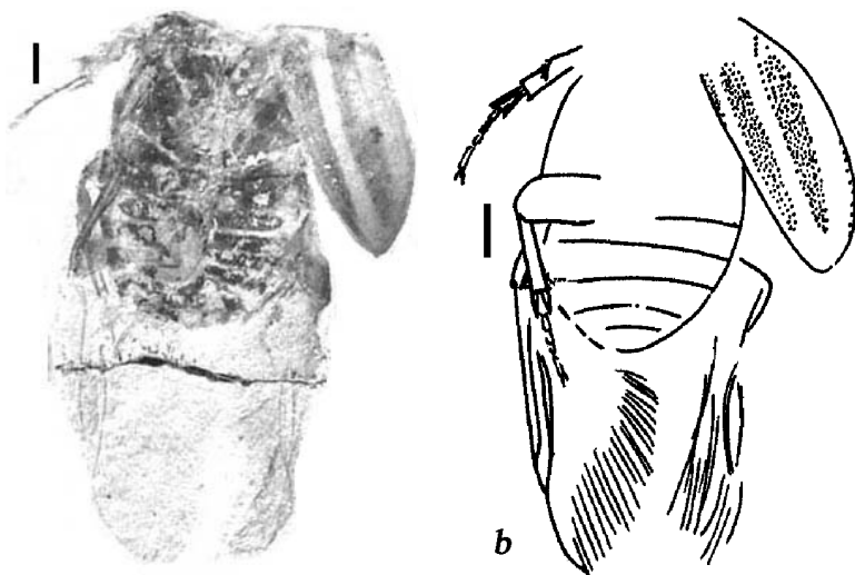
Рис. 56. Antennacrassa picturata (Nikritin), голотип ПИН, № 1989/2994: a – фотография, b – рисунок отпечатка. Прямая линия – 1 мм [По: Никритин, 1977; Николаев, 2004.]
