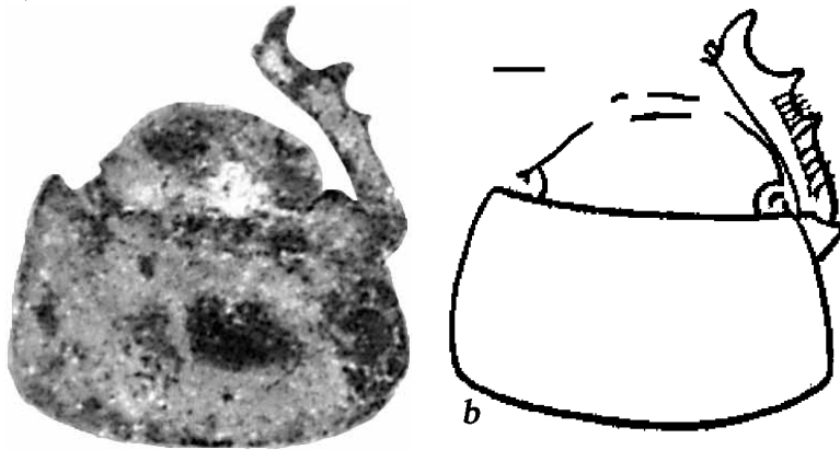
Рис. 70. Lithanomala sibirica (Ponomarenko, 1990), голотип ПИН № 4085/67: a – фотография, b – рисунок. Прямая линия – 1 мм [По: Пономаренко, 1990 и оригинал]
