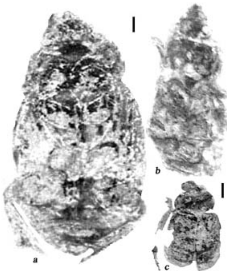
Рис. 52. Виды рода Antemnacrasa Gomez Pallerola: a – A. nigrimontana (Nikolajev), голотип ПИН, № 2904/870; b – A. incerta (Ponomarenko), голотип ПИН, № 4078/11; c – sulcata (Nikritin, 1977), голотип ПИН, № 1668/1785. Прямая линия – 1мм [По: Николаев, 2004]
