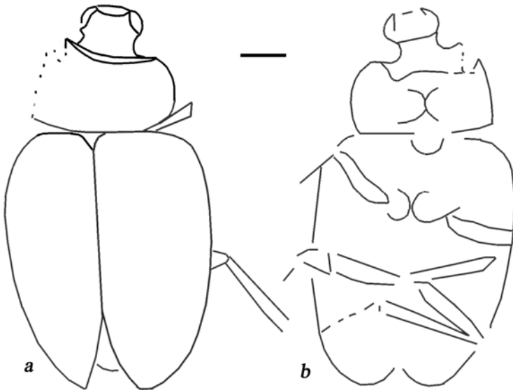
Рис. 24. Leptosorus zherikhini Nikolajev.; голотип ПИН, № 4210/5461 ( a – вид сверху; b – вид снизу). Прямая линия – 1 мм [По: Николаев, 2006]
