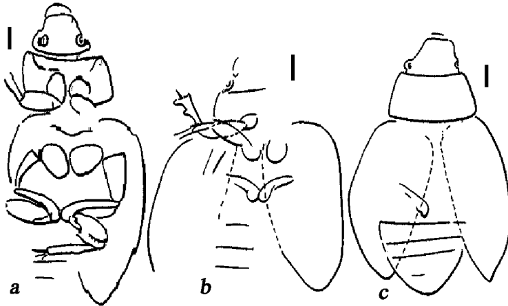
Рис. 62. Antemnacrasa incerta (Ponomarenko): a – голотип ПИН, № 4078/11, b – экземпляр ПИН, № 1742/144, c – экземпляр ПИН, № 1846/85. Прямая линия – 1мм [По: Пономаренко, 1990.]
