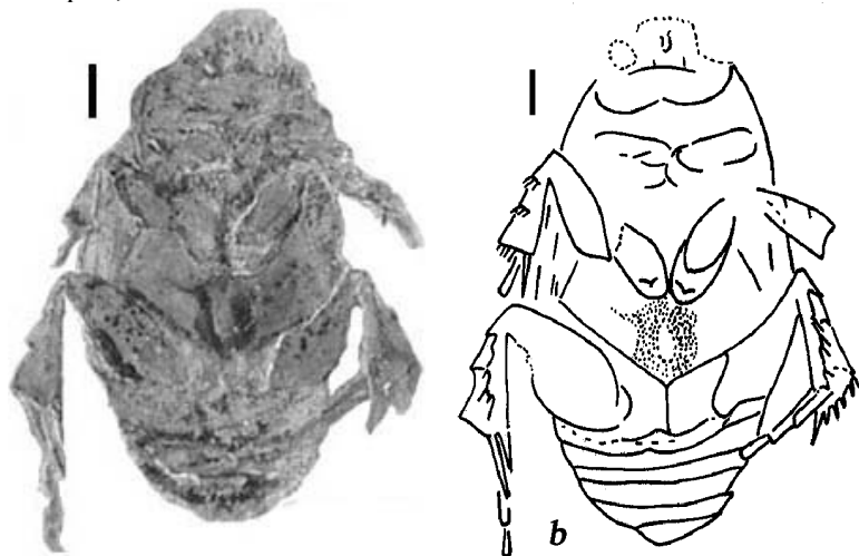
Рис. 60. Antemnacrasa latitibialis (Nikolajev), голотип – ПИН, № 3064/7145: a – фотография, b – рисунок нижней стороны тела. Прямая линия – 1мм [По: Николаев, 1992; 2004.]
