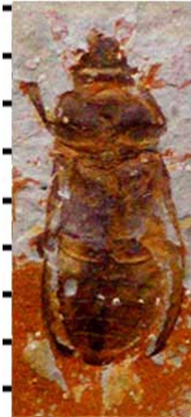
Paralucanus mesosoicus Nikolajev., голотип ПИН, № 4270/1111
