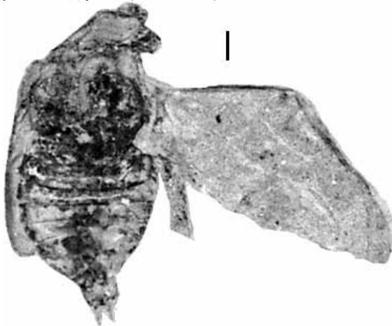
Рис. 7. Cretocoma tologoica Nikolajev голотип ПИН, № 4271/217. Прямая линия - 1 мм
