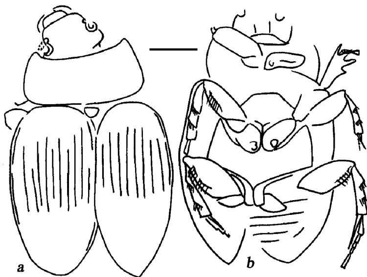
Рис. 57. Antennacrossa sulcata (Nikritin) голотип ПИН, № 1668/1785: a – сверху, b – снизу. Прямая линия – 1мм [По: Никритин, 1977.]
