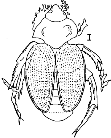
Рис. 5. Proteroscarabaeus yeni Grabau [По: Grabau, 1923]
