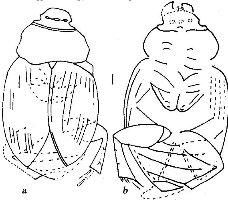
Рис. 53. Antemnacrossa nigrimontana (Nikolajev), голотип ПИН, № 2904/870: a – сверху, b – снизу. Прямая линия – 1мм [По: Николаев, 1992]
