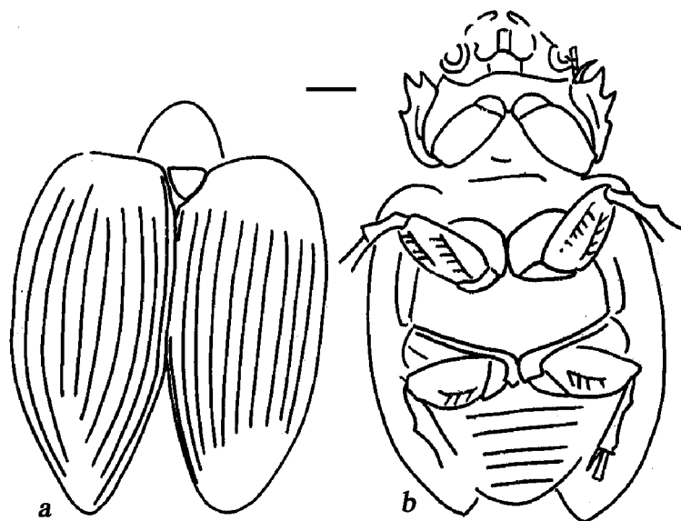
Рис. 58. Antemnacrossa vitimensis (Nikritin) голотип ПИН, № 1668/1805: a – сверху, b – снизу. Прямая линия – 1мм [По: Никритин, 1977.]
