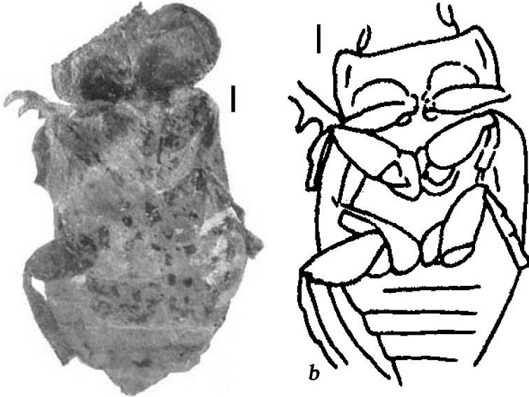
Рис. 61. Antemnacrasa punctata (Ponomarenko), голотип ПИН, № 3149/978: a – фотография, b – рисунок нижней стороны тела. Прямая линия – 1мм [По: Пономаренко, 1986; Николаев, 2004.]
