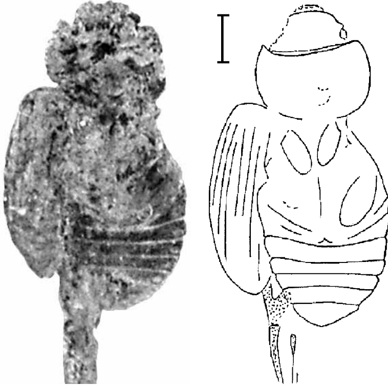
Рис. 40. Cretaegialia aphodiiiformis Nikolajev, 1993, голотип ПИН, № 4210/710: a – фотография, b – рисунок. Прямая линия – 1мм [По: Nikolajev, 1993 и оригинал.]
