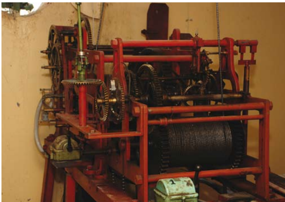
Laikrodžio mechanizmas
