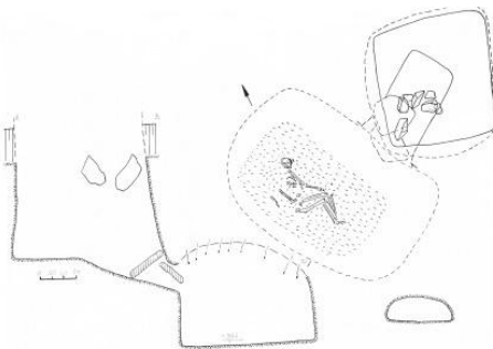
План і розріз пох. 2 вул. Ватутіна, к. 2, 1984
