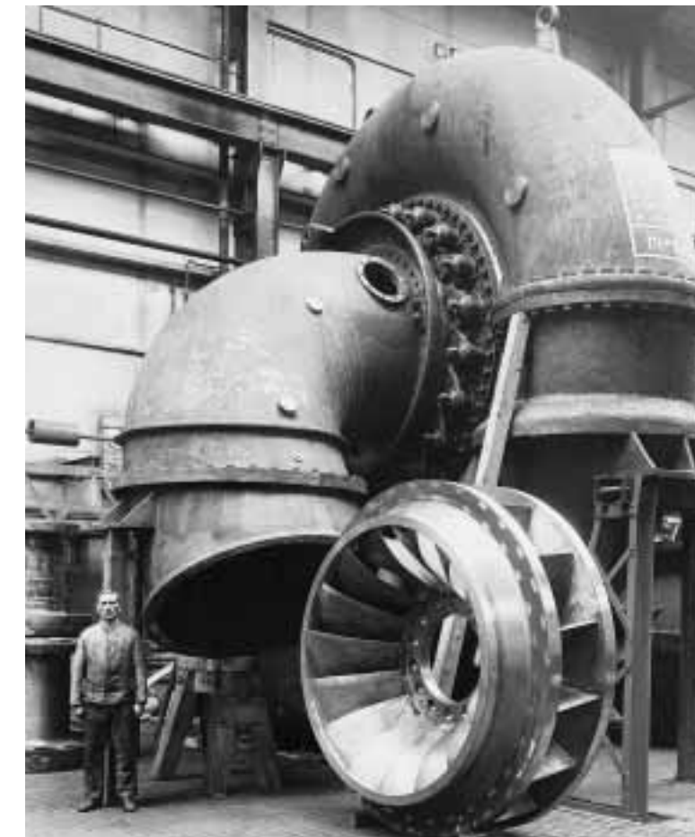
Einbau eines Schaufelrads in eine der vier Pumpen
