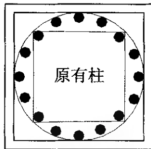
图4 方形截面柱配筋图
