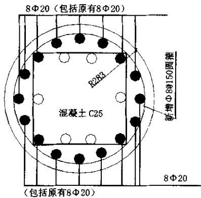
图3 圆形截面柱配筋图
