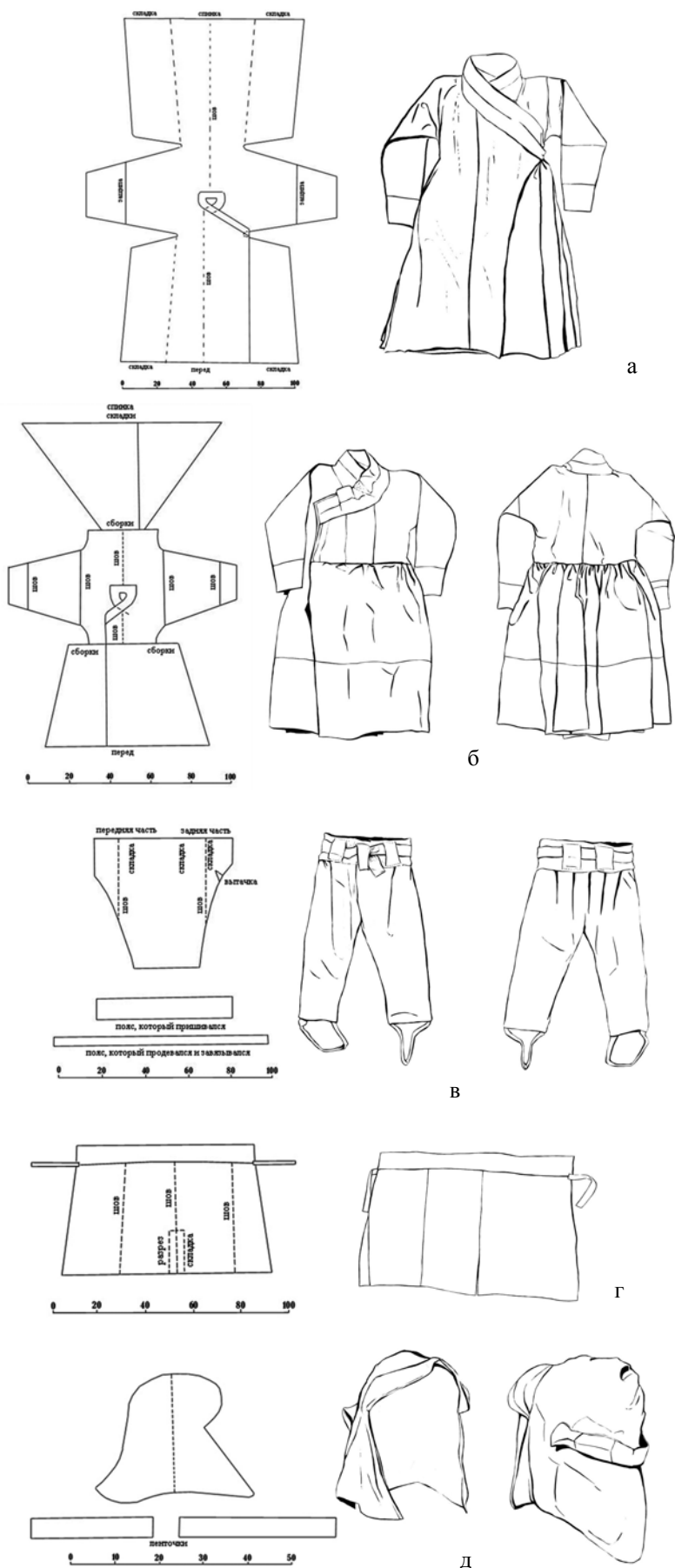
Схема 3. Одежда мальчика из погребения 3 на горе Окошки (выкройки по Т.Н. Никитиной): а – утепленный халат; б – основной халат; в – штаны; г – «набрюшник»; д – головной убор.
