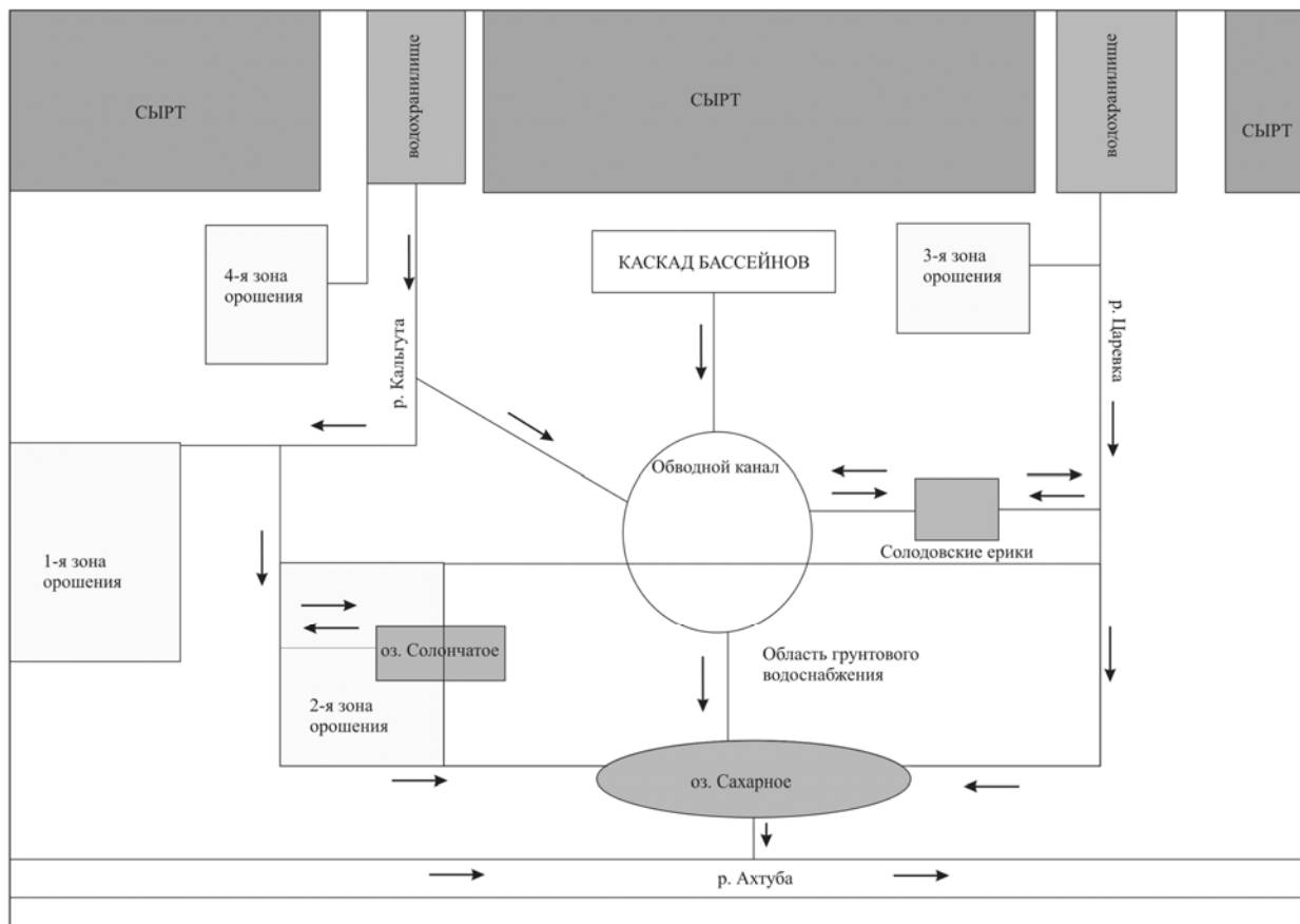
Рис. 13. Принципиальная схема водоснабжения Царевского городища.
