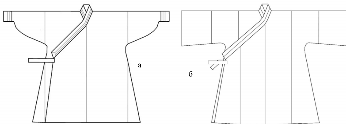
Схема 2. «Большие» женские халаты: а – общая схема (один из вариантов) «большого» халата с суживающимися к запястьям рукавами; б – общая схема (один из вариантов) «большого» халата с широкими рукавами
