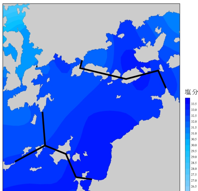
図 8-2 上層の塩分分布
