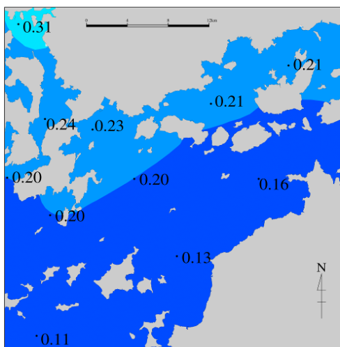
図 8-16 安芸灘における上層の TN、TP 分布
