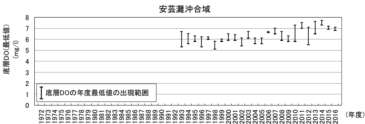
図 8-21 公共用水域水質測定地点及び底層 DO 年度最低値の出現範囲の推移
