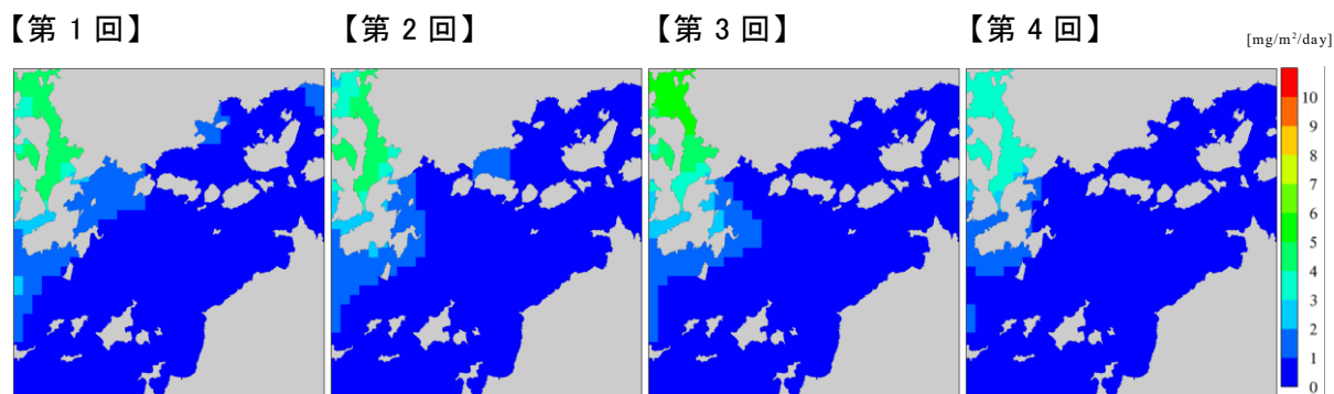
図 8-27 安芸灘におけるりん溶出量(年平均値)の状況
