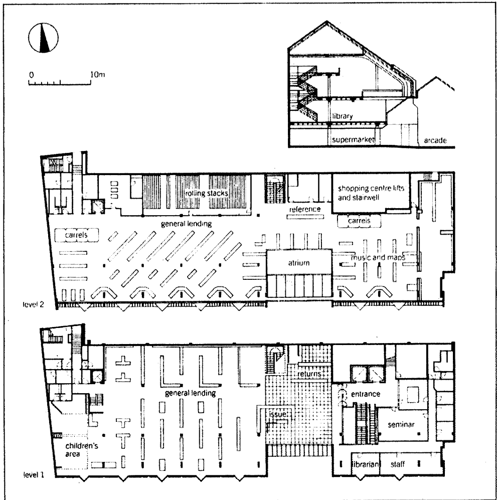
▲圖二 設計平面圖
