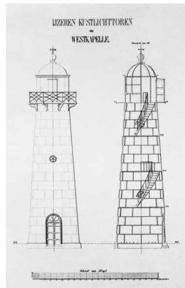
Bouwtekening uit 1875.
