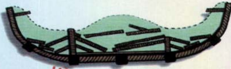
رسم تفصيلي لهيكل السفينة من الداخل
