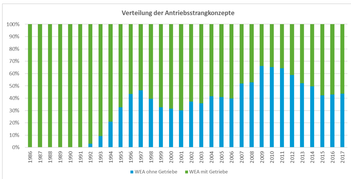
Abbildung 53: Anteile der Antriebskonzepte (bezogen auf die Nennleistung der Neuinstallationen) als Funktion des Jahres der Inbetriebnahme
