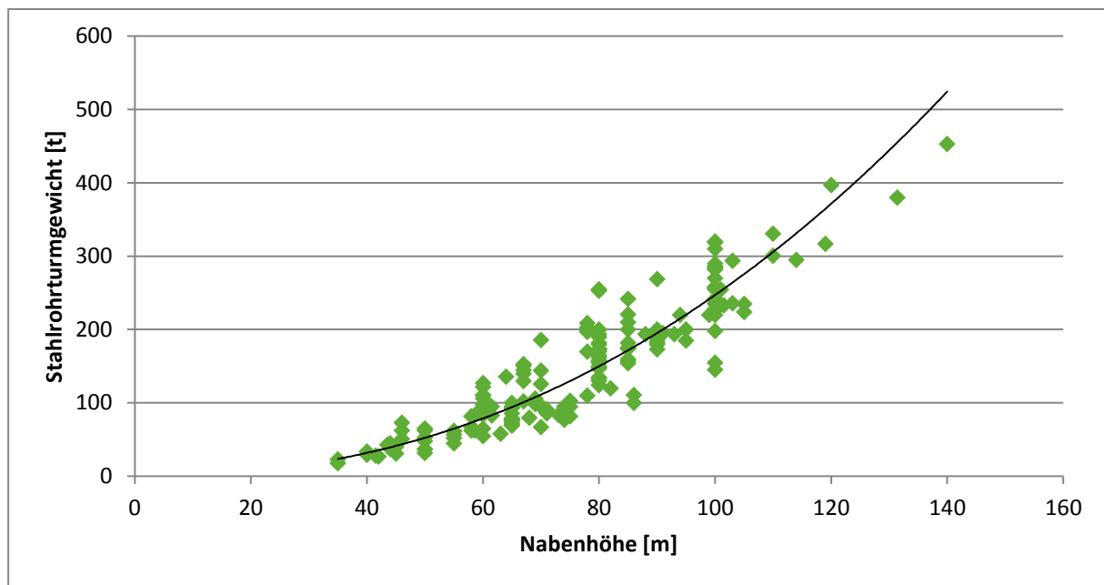
Abbildung 47: Stahlrohrturmgewichte [t] als Funktion der Nabhöhe [m]
