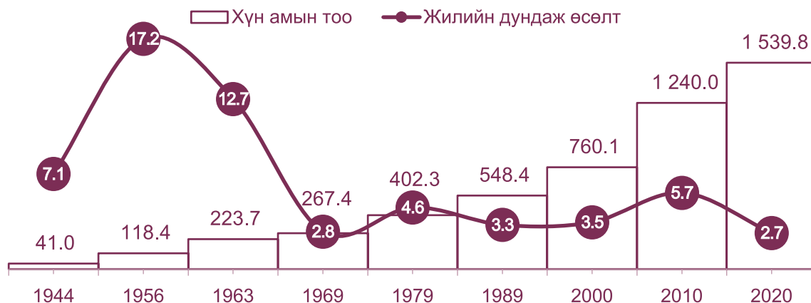
ЗУРАГ 2.2. ХҮН АМЫН ТОО, ТООЛЛОГО ЯВАГДСАН ОНУУДААР*
