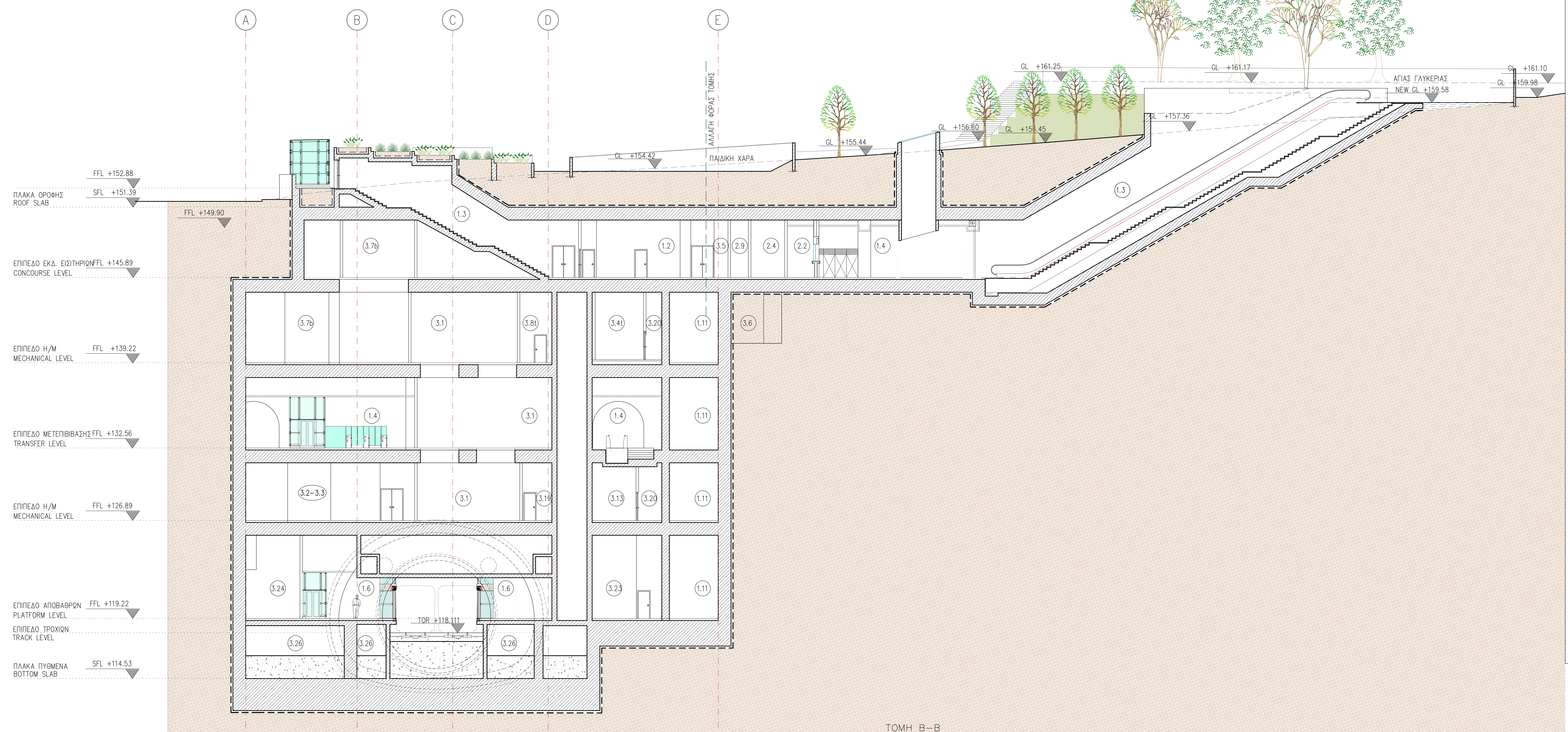
TOMH B-B
