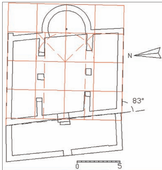
Fig. 102 - Santa Croce Camerina, Basilica di Kaukana. Pianta: lettura progettuale
