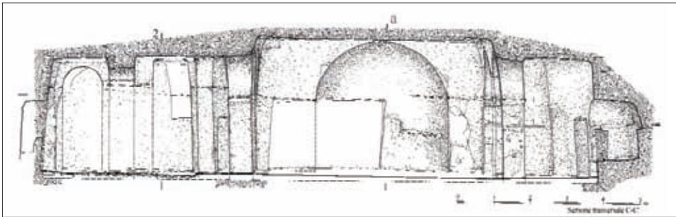
Fig. 92 - Basilica. Sezione longitudinale d-d'
