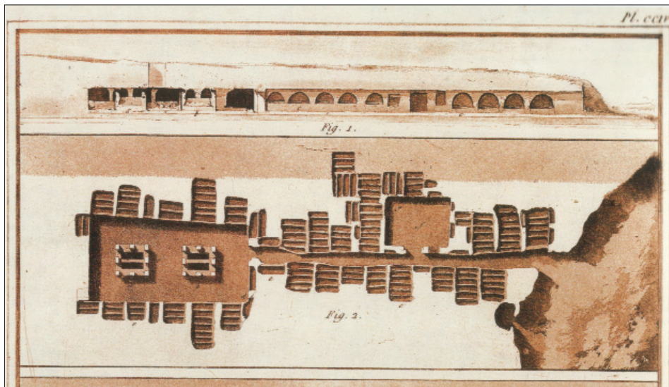
Fig. 14 - J.L. Hoüel. Ipogeo I di Stafenna (Rosolini). Pianta e sezione
