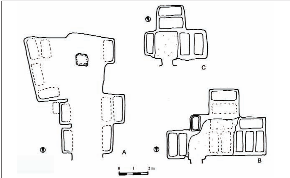
Fig. 59 - Cava Grande, Croce Santa/ Zacco Miccio. Piante degli ipogei
