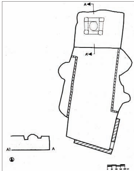
Fig. 54 - Cava Grande, Cansisini. Planimetria e sezione longitudinale del recesso con baldacchino dell'ipogeo B
