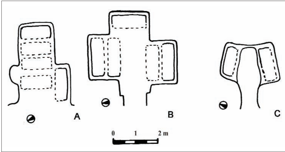
Fig. 55 - Cava Grande, Zacco Miccio. Piante degli ipogei
