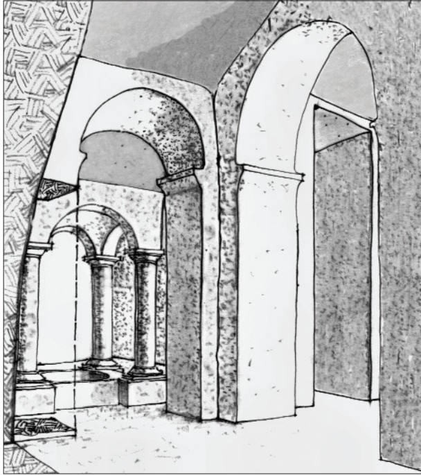
Fig. 118 - Basilica. Vani B e C. Restituzione
