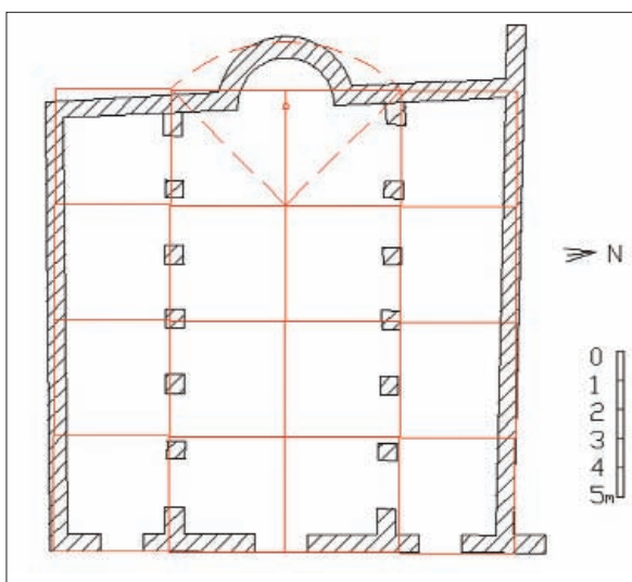
Fig. 100 - Salemi, Basilica di S. Miceli. Pianta: lettura progettuale
