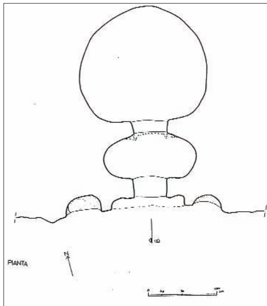
Fig. 25 - C.da Granati Vecchi. Tomba a fronte pilastrata. Pianta
