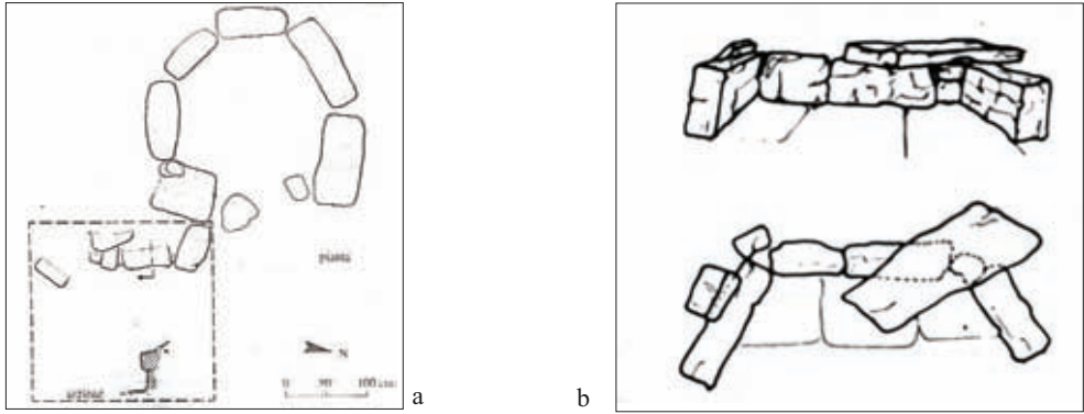
Fig. 29 Cava dei Servi a) "dolmen" 1. Pianta b) "domen" 2. Alzato prospettico e pianta
