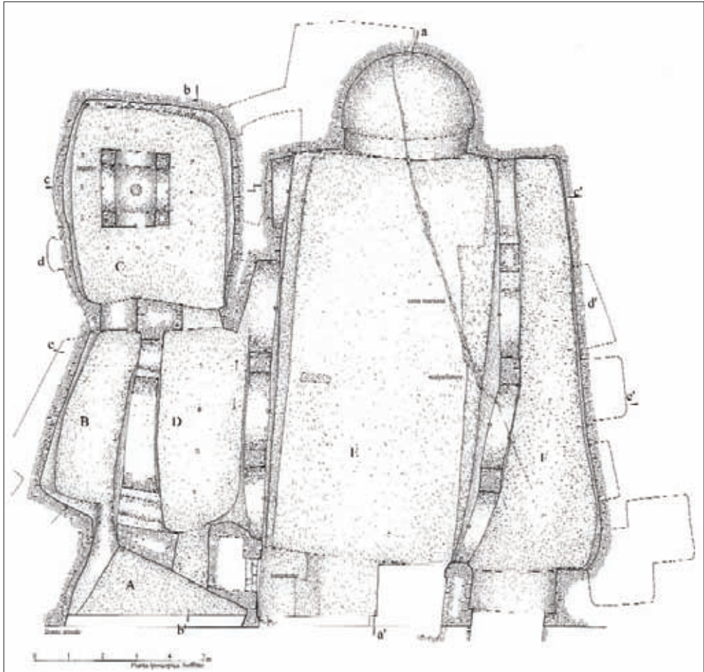
Fig. 75 - Basilica. Pianta iposcopica
