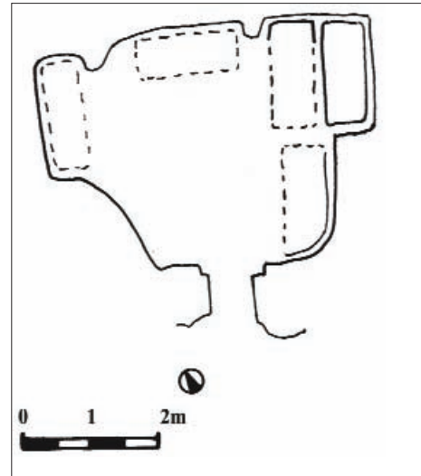
Fig. 38 - Cava Prainito. Pianta dell'ipogeo
