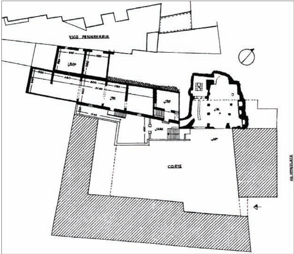
Fig. 72a - Palazzo Platamone. Pianta del piano terreno
