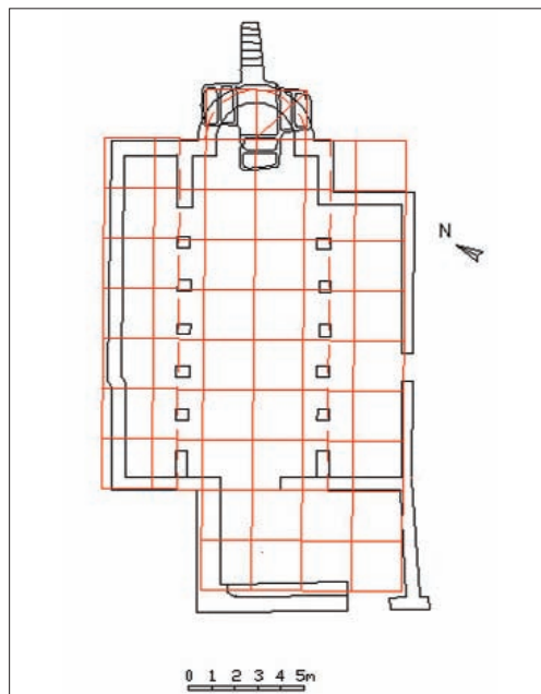
Fig. 106 - Cittadella, Basilica martiriale. Pianta: lettura progettuale
