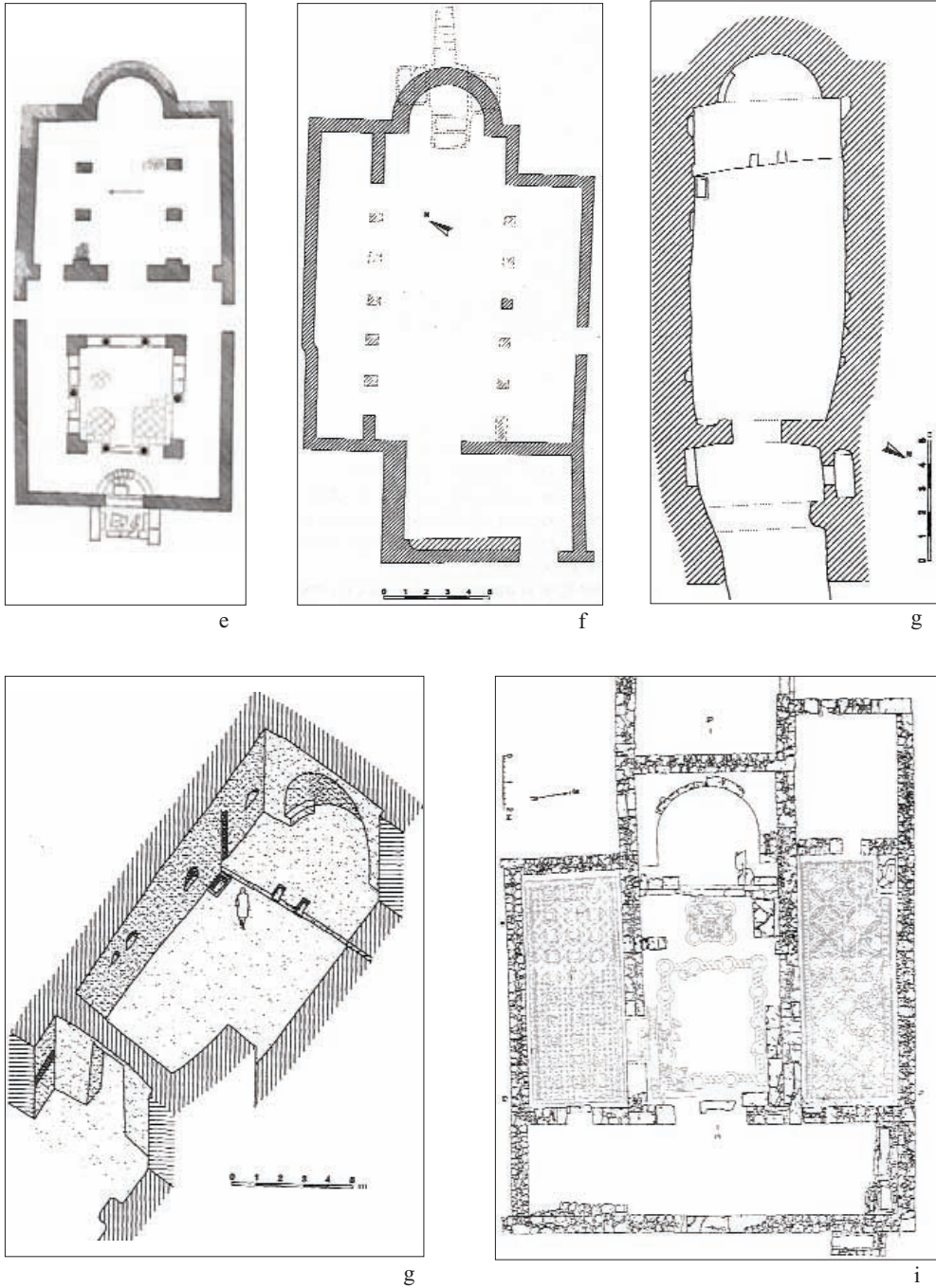
Fig. 130e-i - Basiliche cristiane della Sicilia: e) Monte Po (da LIBERTINI 1928, fig. 2); f) Cittadella (da GIGLIO 2003, p. 13); g) Bibinello. Pianta e assonometria (da GIGLIO 2003, pp. 137-138); h) Pirrera (da BONACASA CARRA 1999, fig. 8).
