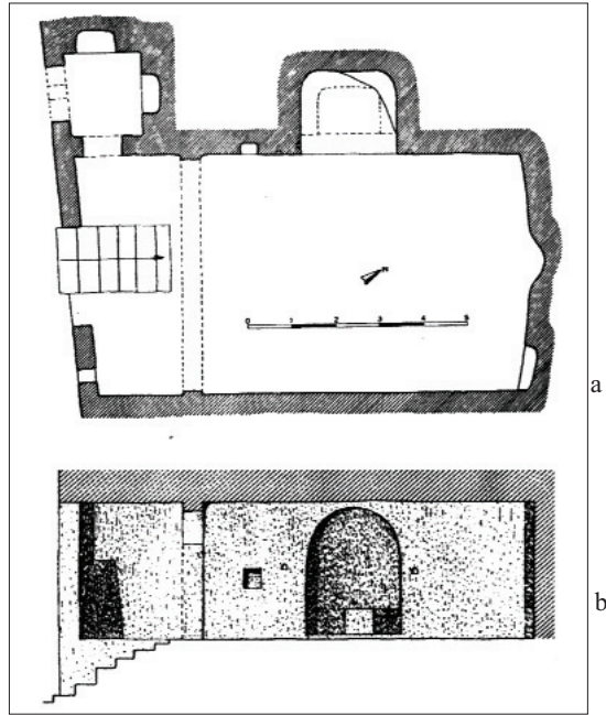
Fig. 53 a - Cava Grande, Cansisini, chiesa rupestre. a) Planimetria; b) sezione longitudinale
