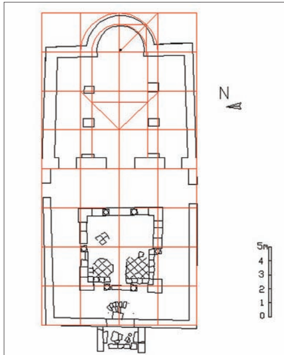
Fig. 101 - Catania, Basilica di Monte Po. Pianta: lettura progettuale
