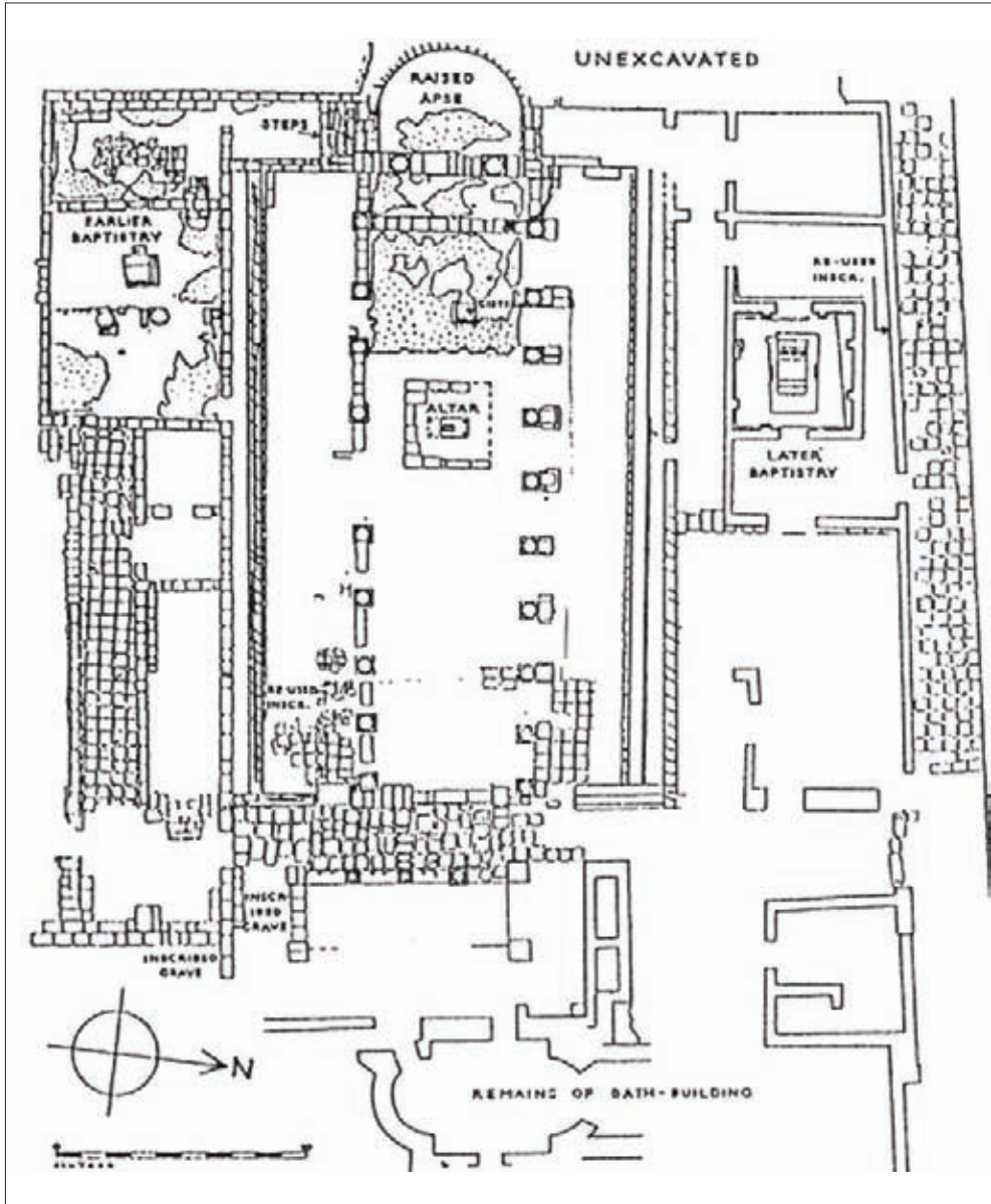
Fig. 109 - Sabratha, Basilica cristiana del foro. Pianta
