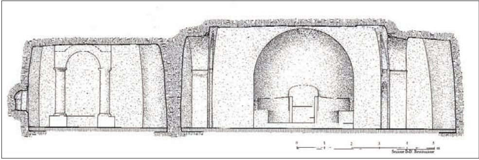
Fig. 126 - Basilica. Sezione trasversale di restituzione, c-c'
