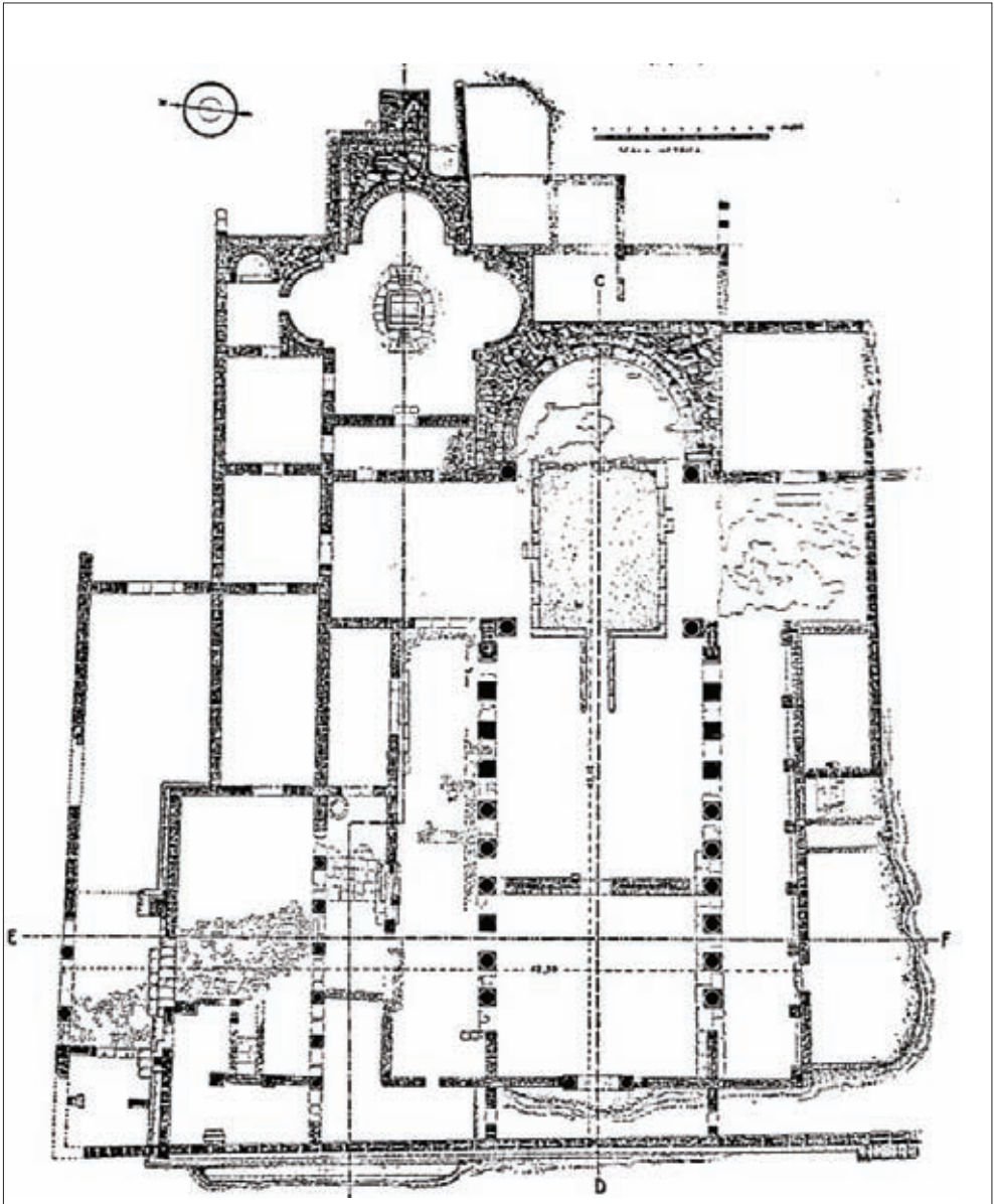
Fig. 110 - Apollonia, Basilica. Pianta
