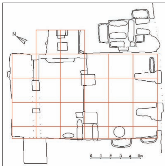
Fig. 108 - Buscemi, Basilica rupestre di S. Pietro. Pianta: lettura progettuale
