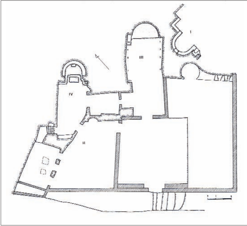
Fig. 116 - Rosolini. Grotta di Croce Santa. Pianta
