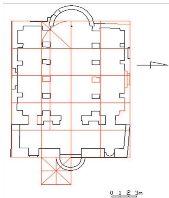
Fig. 104 - Siracusa. S. Pietro intra moenia. Pianta: lettura progettuale
