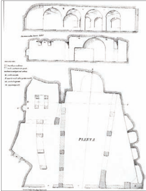
Fig. 73 - Basilica. Sezioni e pianta (da Sciuto Patti)
