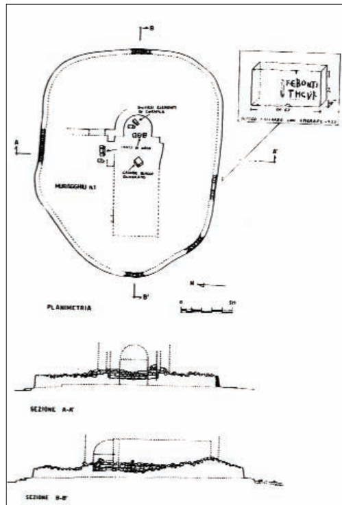
Fig. 41 - Cava Prainito, Cozzo Tondo. Planimetria dei resti della chiesa inglobati nel "muragghiu"
