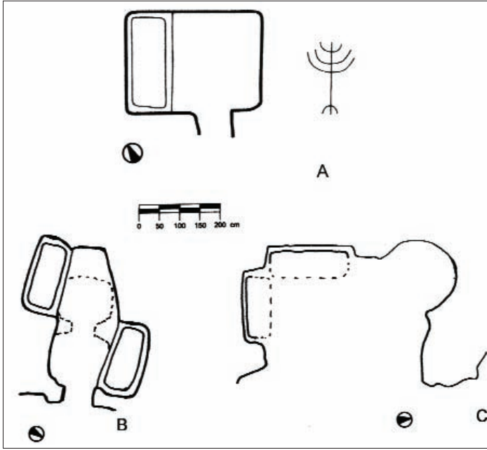
Fig. 50 a-c – Cava Grande, Pernice. Piante degli ipogei
