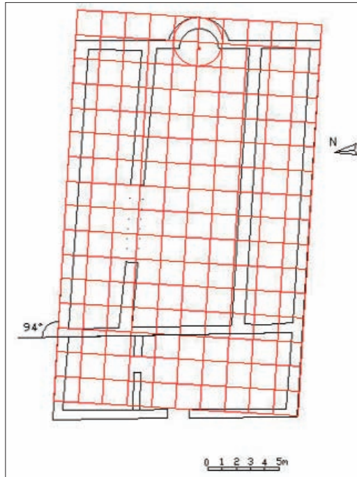
Fig. 105 - Eloro, Basilica. Pianta: lettura progettuale
