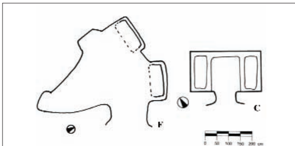
Fig. 44 - Cava Prainito, Mulino Grotte. Pianta degli ipogei
