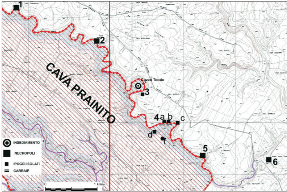
Fig. 37 - Cava Prainito. Planimetria generale con indicazione dei siti citati (stralcio da C.T.R. 1:10000)
