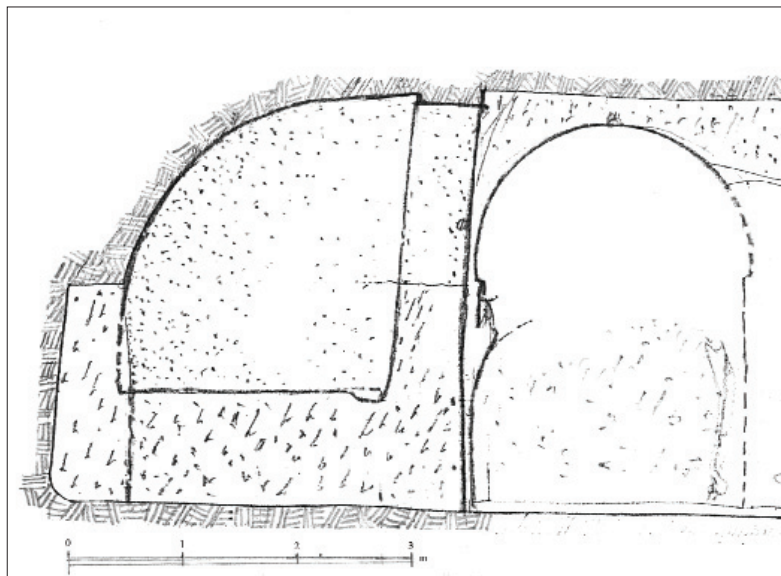
Fig. 89 - Basilica. Conca absidale, sezione
