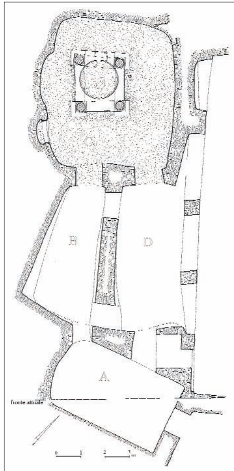
Fig. 127 - Basilica. Annesso catecumenale: vani A-D. Pianta
