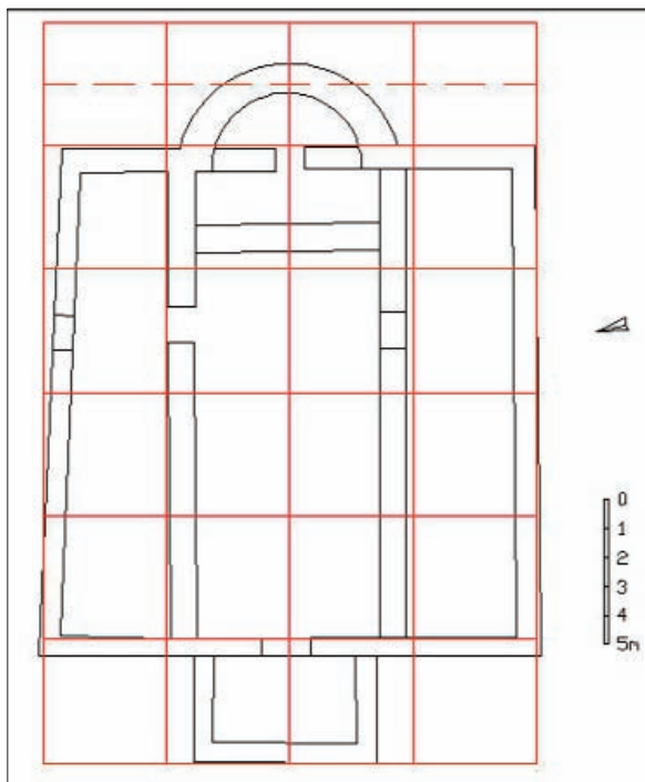
Fig. 99 - Piazza Armerina, Basilica di Sofiana. Pianta: lettura progettuale
