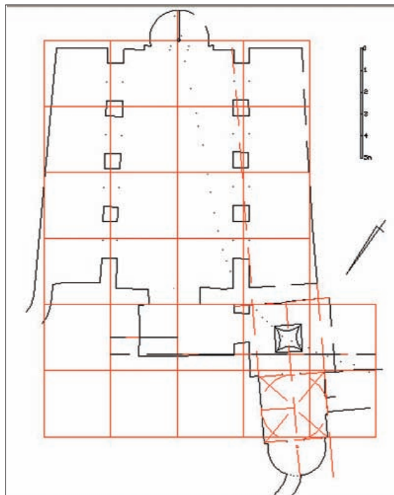
Fig. 107 - Noto, Basilica rupestre di S. Marco. Pianta: lettura progettuale
