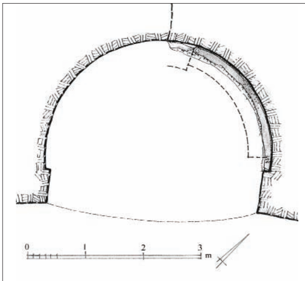
Fig. 88. - Basilica. Conca absidale, pianta
