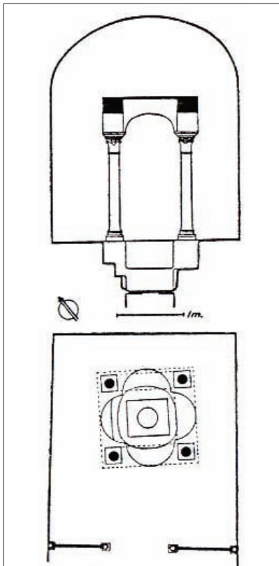
Fig. 121h - Battisteri con teguri tetrastili: e) Leptis Magna 4 (241); f) Qued Ramel (239); g) Cartagine Sayda (275b); h) Hippona, grande basilica (da MAREC 1958, p. 103, fig. 2).
