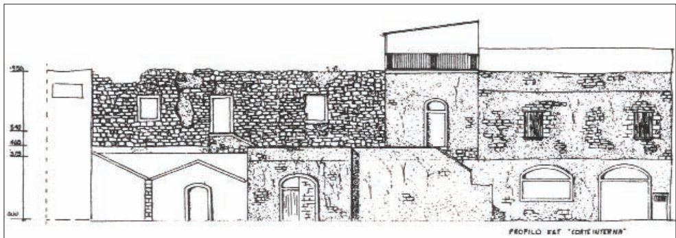
Fig. 72b - Palazzo Platamone. Fronte sulla corte
