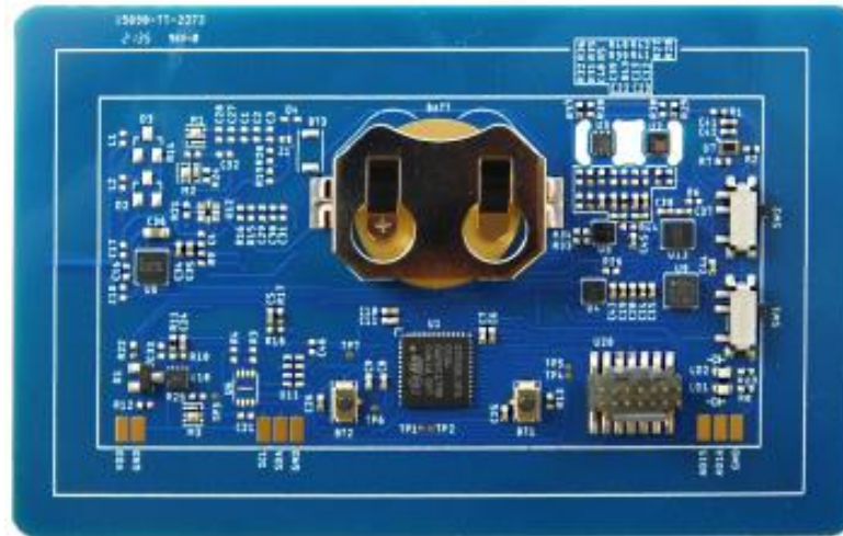
STEVAL-SMARTAG2
