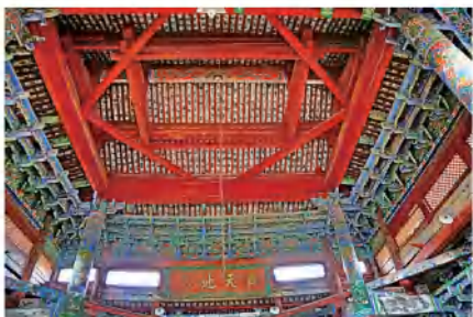
先师庙栝梁结构
