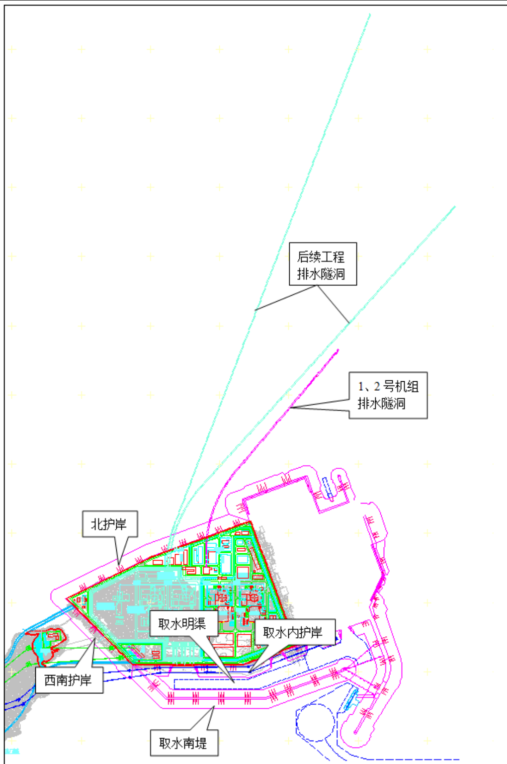
图 6.1-1 取排水工程方案平面布置图
