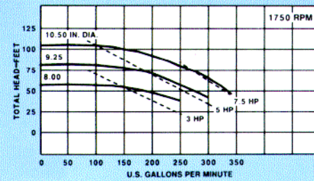
PV 4 x 4 x 8A
