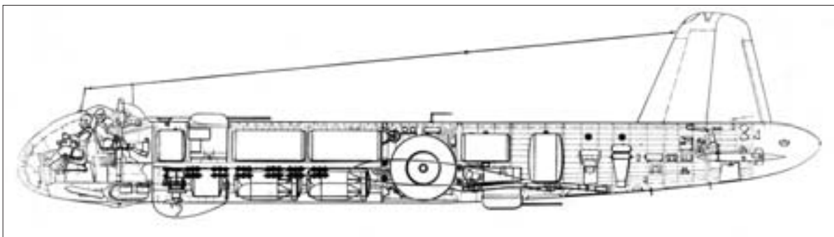
Компоновка фюзеляжа «140-Б/Р»
