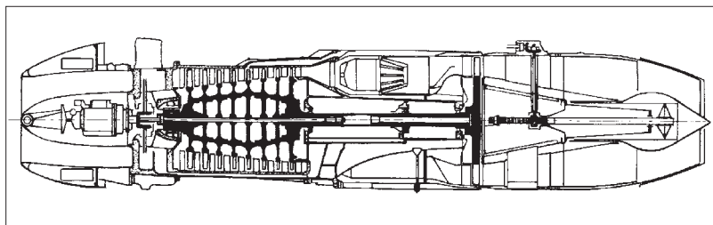
Схема двигателя BMW 003
