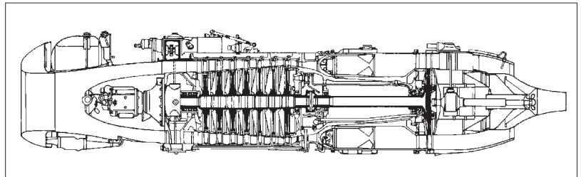
Схема двигателя Jumo 004В
