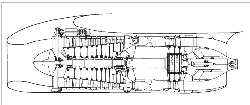
Схема двигателя BMW 018
