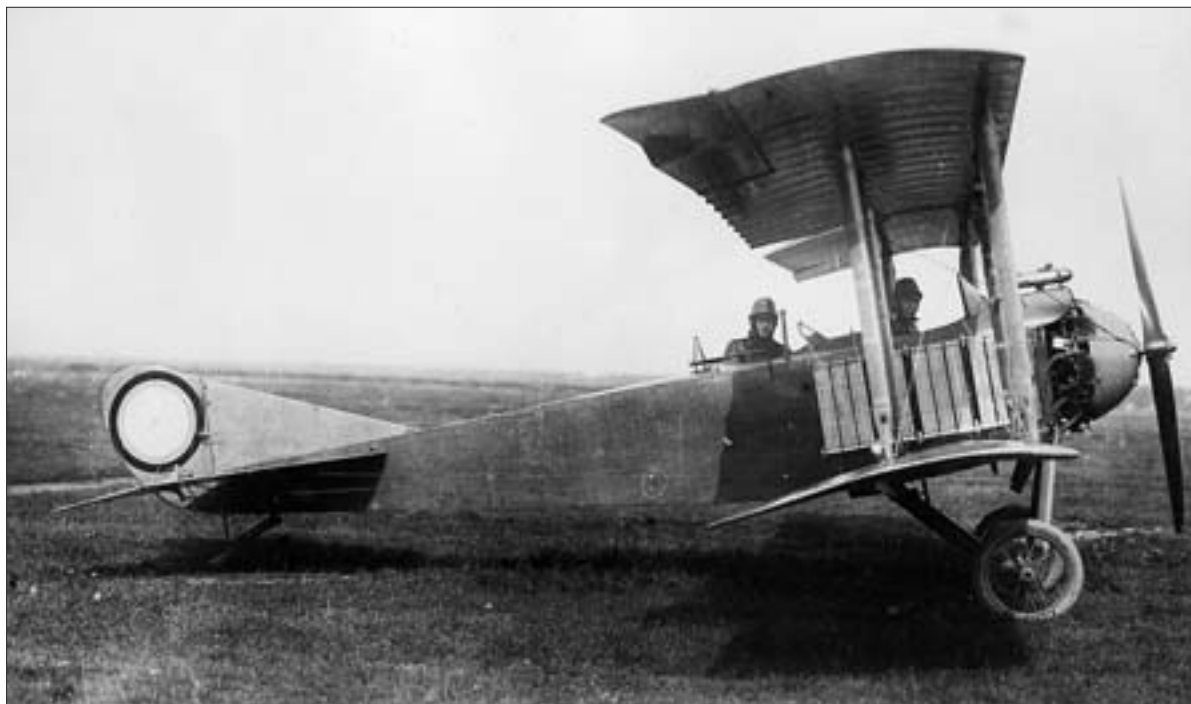
«Лебедь-ХІІ» с двигателем «Сальмсон», заводской № 457. Комендантский аэродром, 1916 г.
