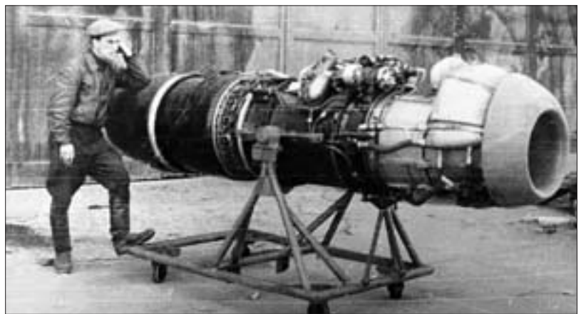
Один из двигателей Jumo 004, найденных советскими войсками в Австрии
