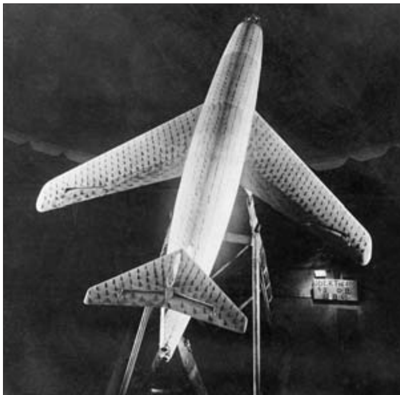
Исследование самолета «346» в аэродинамической трубе ЦАГИ
