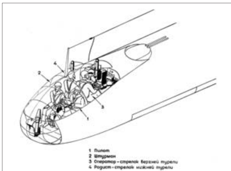
Компоновка кабины экипажа «140-Р»
