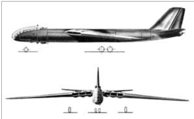
Проектный рисунок тяжелого бомбардировщика EF 132
