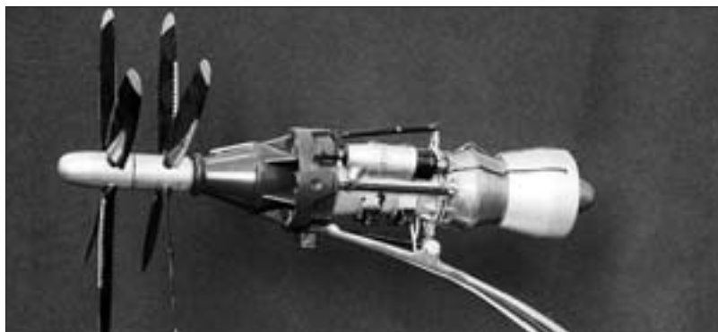
Модель двигателя НК–12
