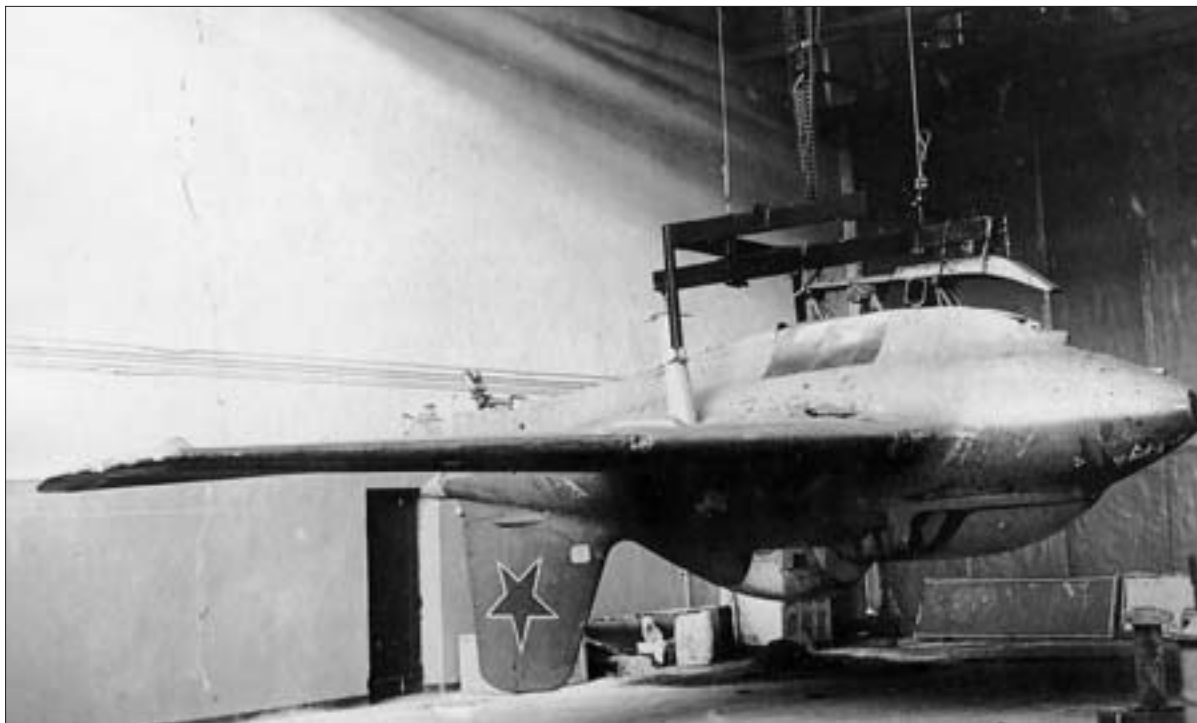
Me 163S на статиспытаниях в ЦАГИ
