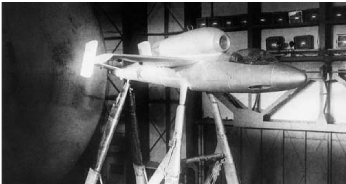
Самолет He 162 в аэродинамической трубе Т-101 ЦАГИ
