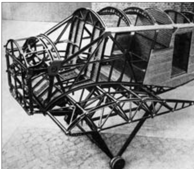
Каркас самолета Юнкерс F 13
