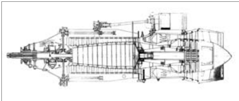
Схема турбовинтового двигателя «022»
