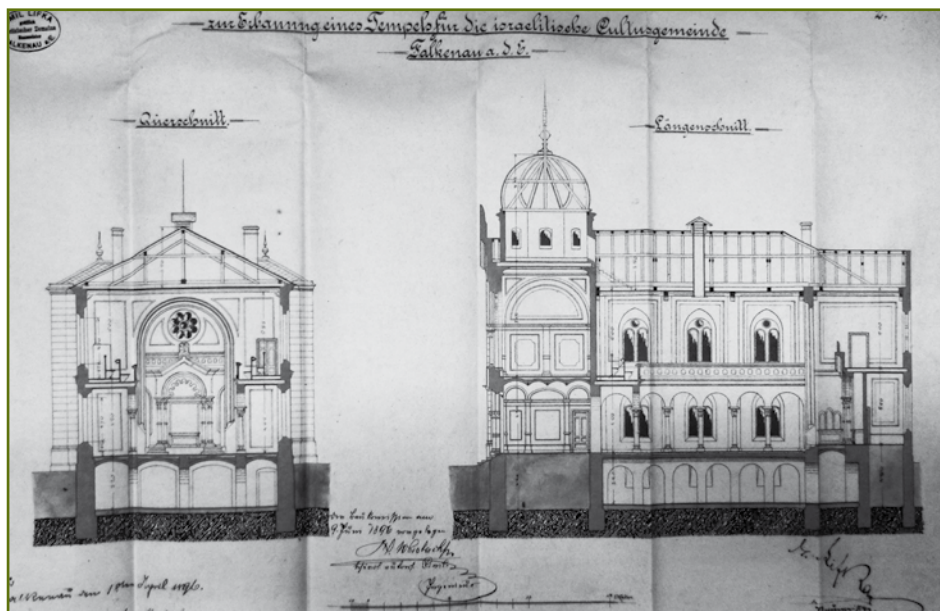
Řezy budovou.
