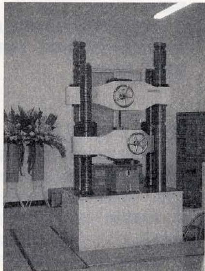
材料試驗中心的萬能試驗機。
