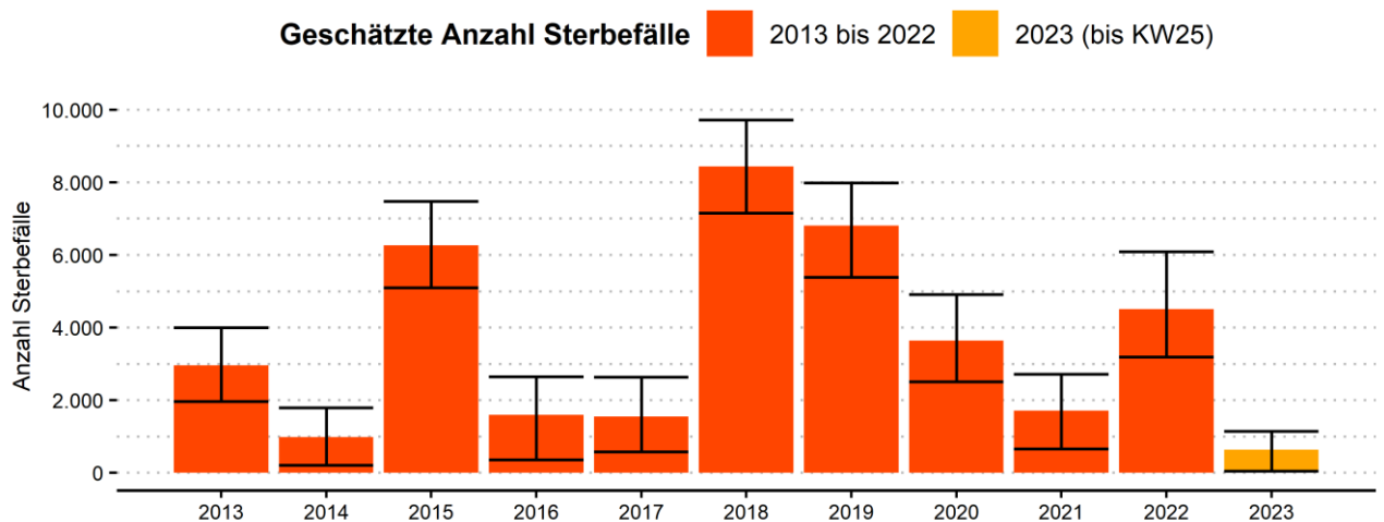
Abbildung 3. Geschätzte Anzahl hitzebedingter Sterbefälle im Zeitraum 2013 - 2023 in Deutschland. Die Schätzung für das Jahr 2023 ist noch unvollständig.
