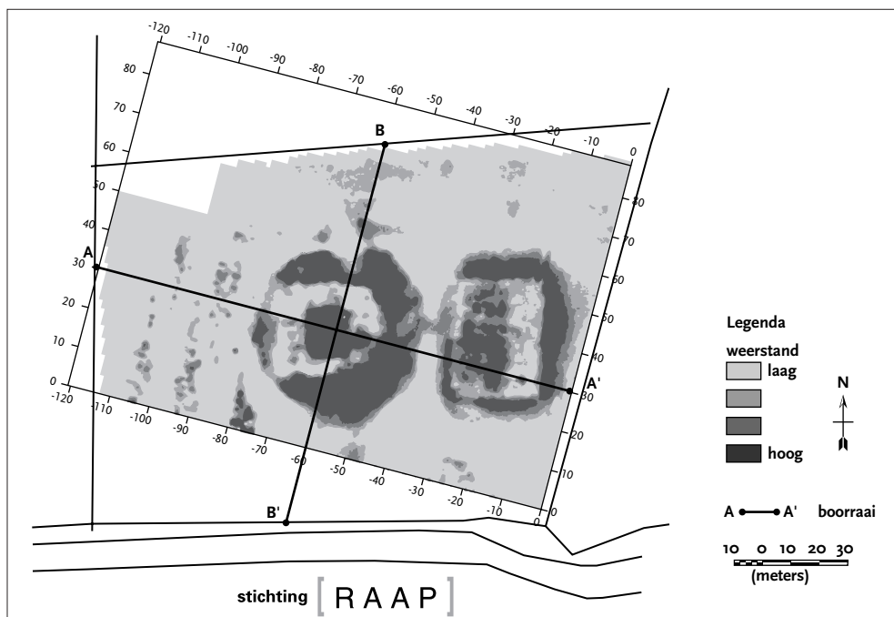
Afb. 7 Resultaten van het weerstandsonderzoek op het terrein van het Kasteel van Selwerd. Tekening: Stichting RAAP, Amsterdam.
