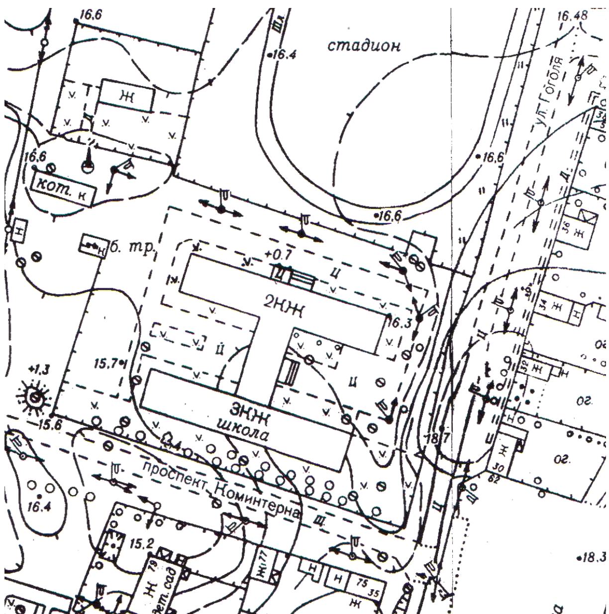
Фрагмент топографического плана масштаба 1:2000
