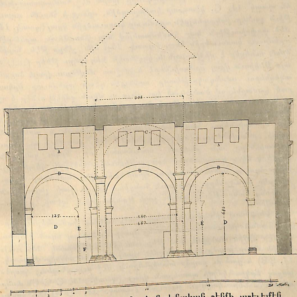
Պատկեր 14. Տեկորի տաճարի նախնական շէնքի արեւելեան արեւմուտքի հասուածականը
