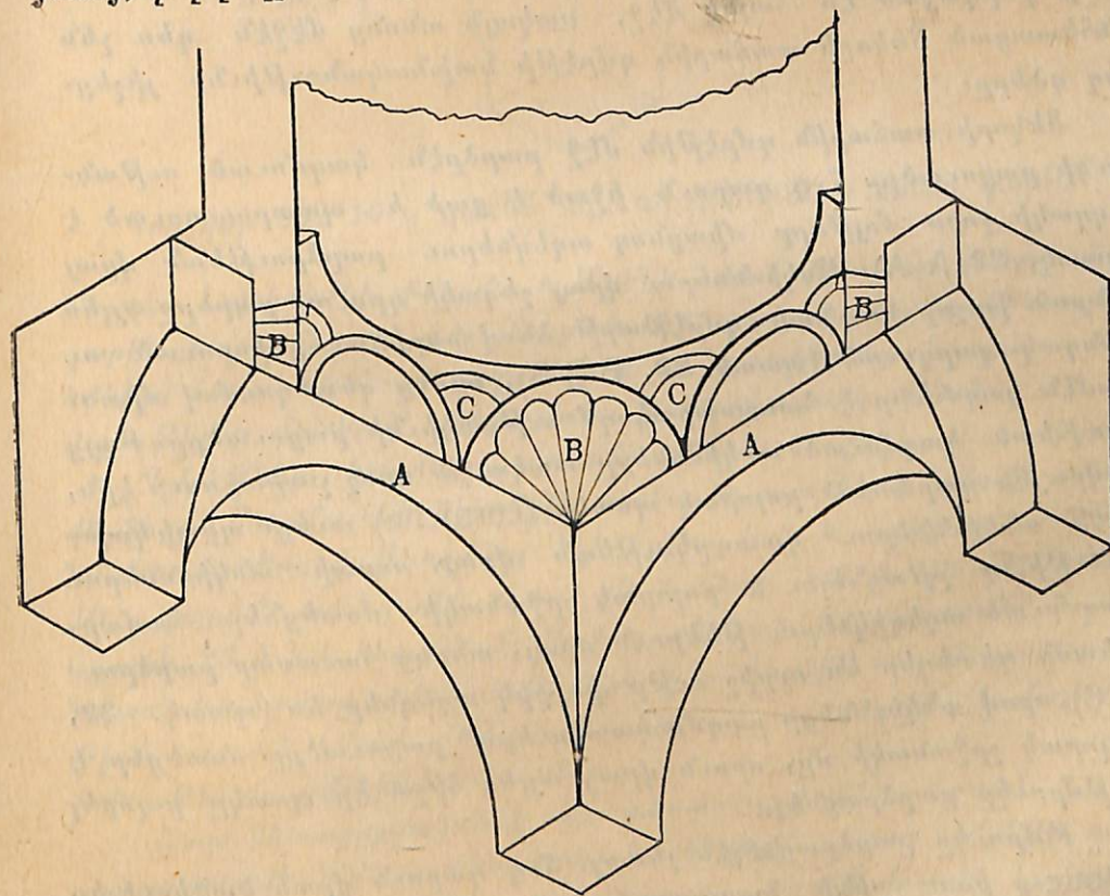
Պատկեր 22. 7-րդ դարէն մինչև 10-դ դարու գմբէթները ներսի կողմէն:
