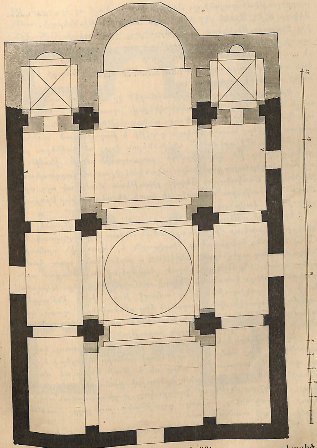
Պատ. 17. Մրենի տաճարի կրած փոփոխութիւնները պարզող յասակագիծ.
