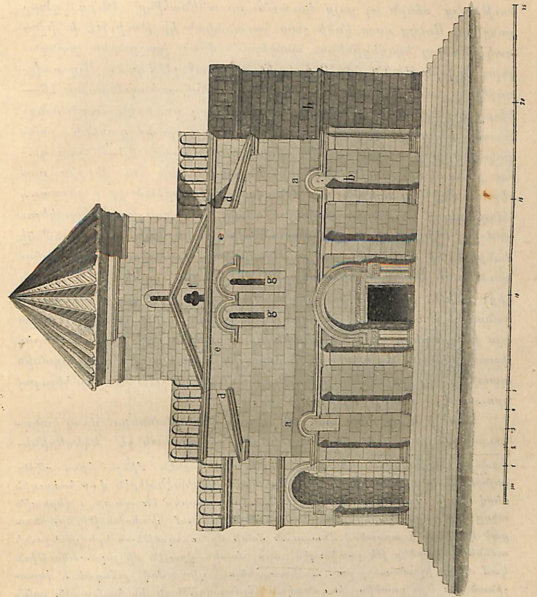
Պատկեր 9. Տեկորի տաճարի արեւմտեան ճակատը
