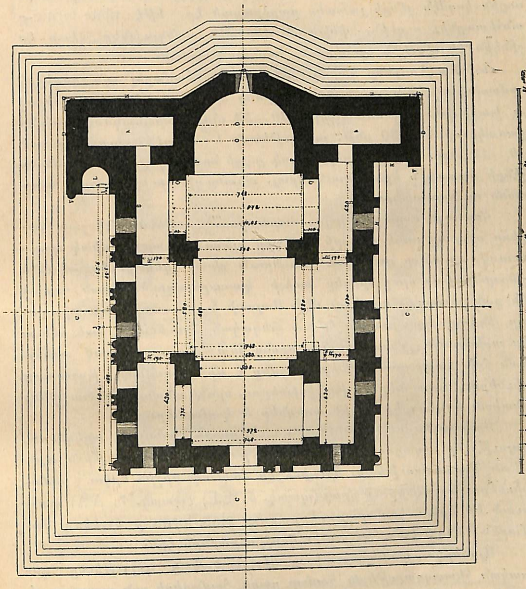
Պատկեր 5-րդ. Տեկորի տաճարի այժմեան յատակագիծը
