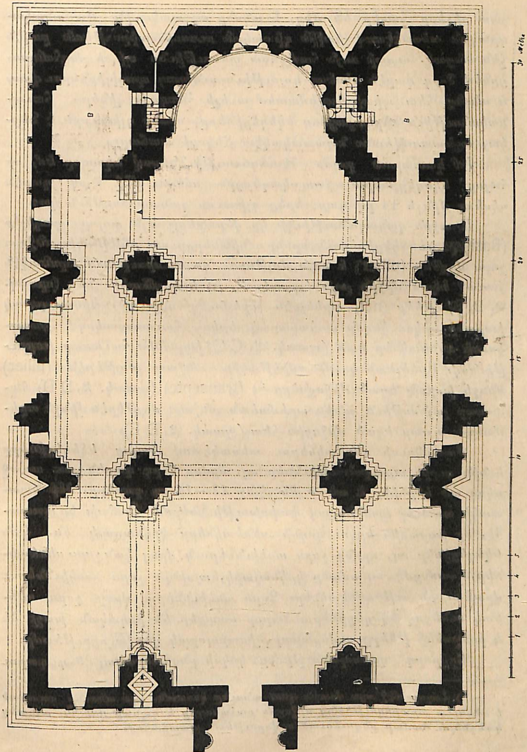
Պատկ. 3. Յասակագիծ Անիի կաթողիկէ մայր եկեղեցւոյ.
