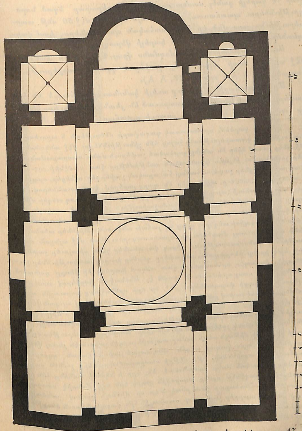
Պատկեր 16. Մրենի տաճարի այժմեան յատակագիծը:
