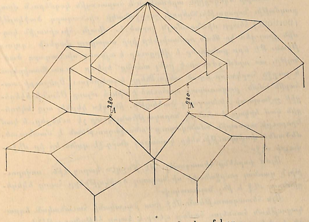
Պատկեր 24. Տեկորի տաճարի գմբեթը
