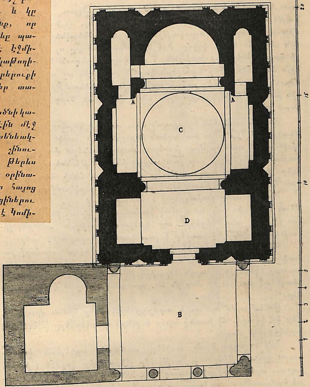
Պատկ. 4-րդ. Յասակազիծ Անիի Ս. Գրիգոր Լուսաւորիչ (Նախւի) եկեղեցիի
