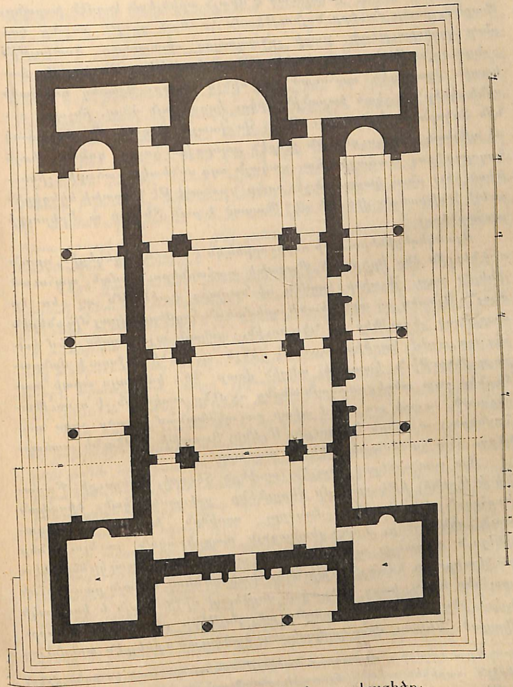
Պատկեր 18. Երեբունքի տաճարի յատակադիծը:
