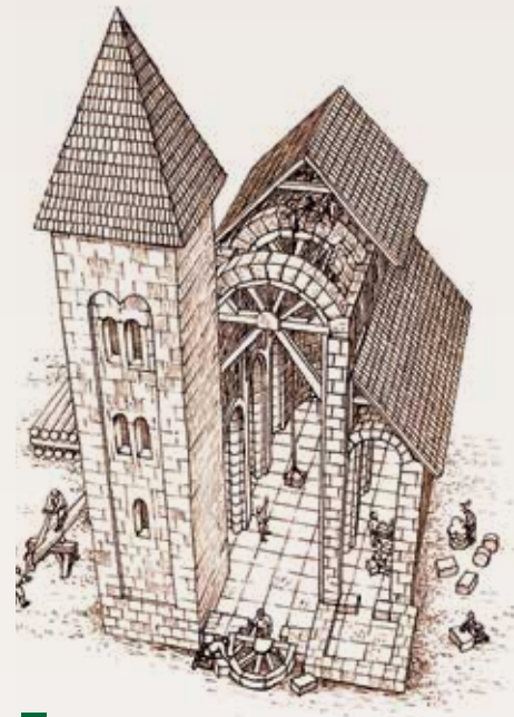
Így épült a román stílusú templom
