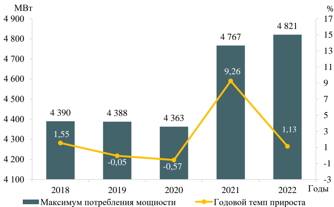
Рисунок 3 – Максимум потребления мощности энергосистемы Республики Татарстан и годовые темпы прироста
