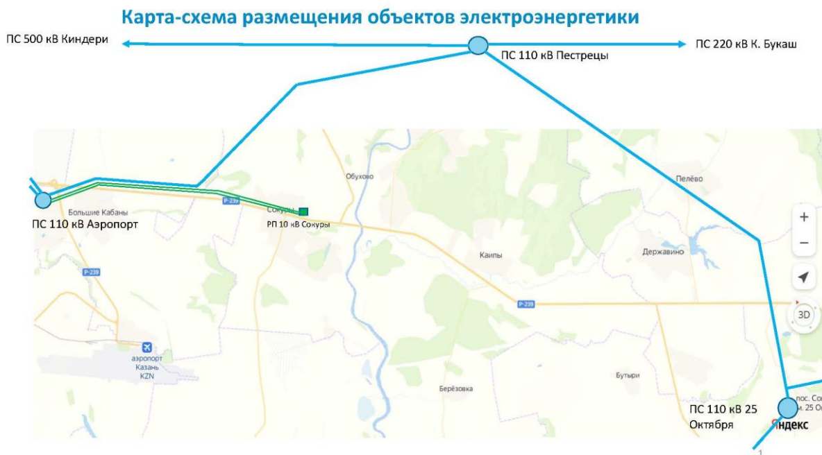
Рисунок 4 – Карта-схема электрических сетей энергорайона размещения РП 10 кВ Сокуры
