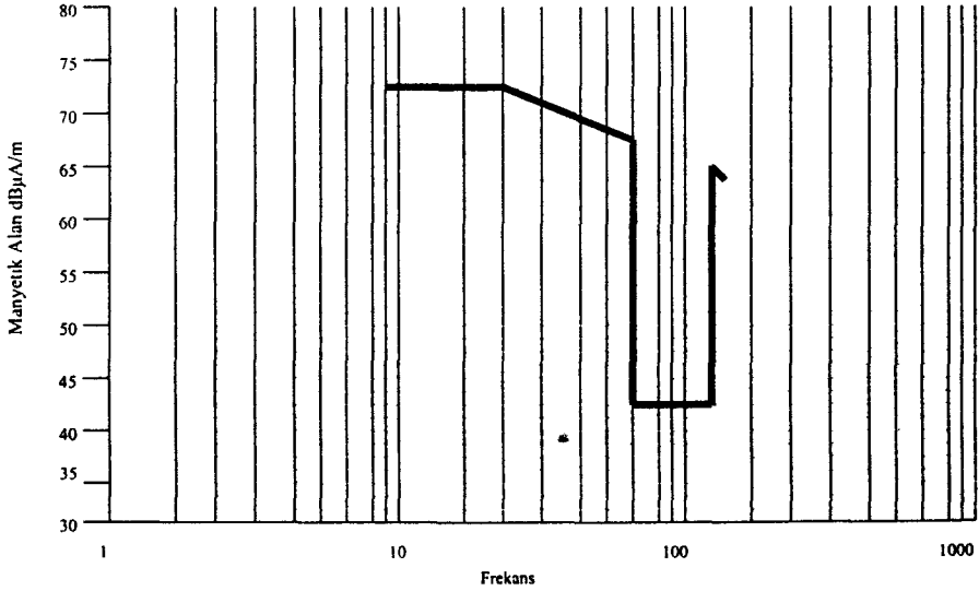
Şekil 1 - 9-135 kHz aralığında 10 metrede ölçülen manyetik alan limitleri
